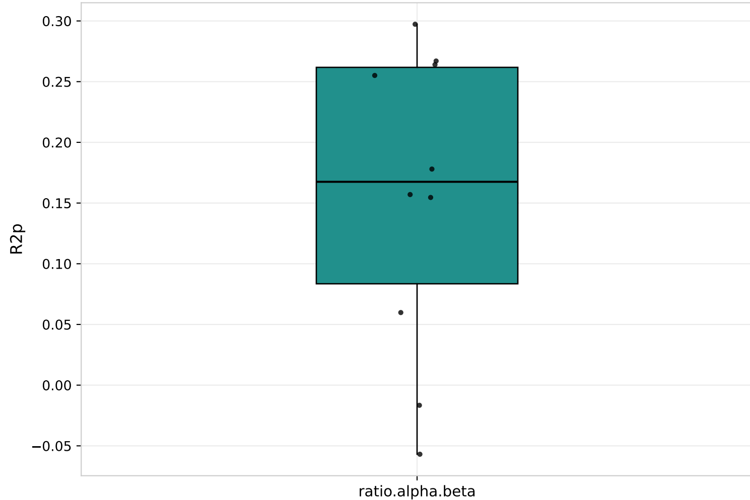
Boxplot des R2p obtenus pour ratio.alpha.beta sur les 10 iterations
