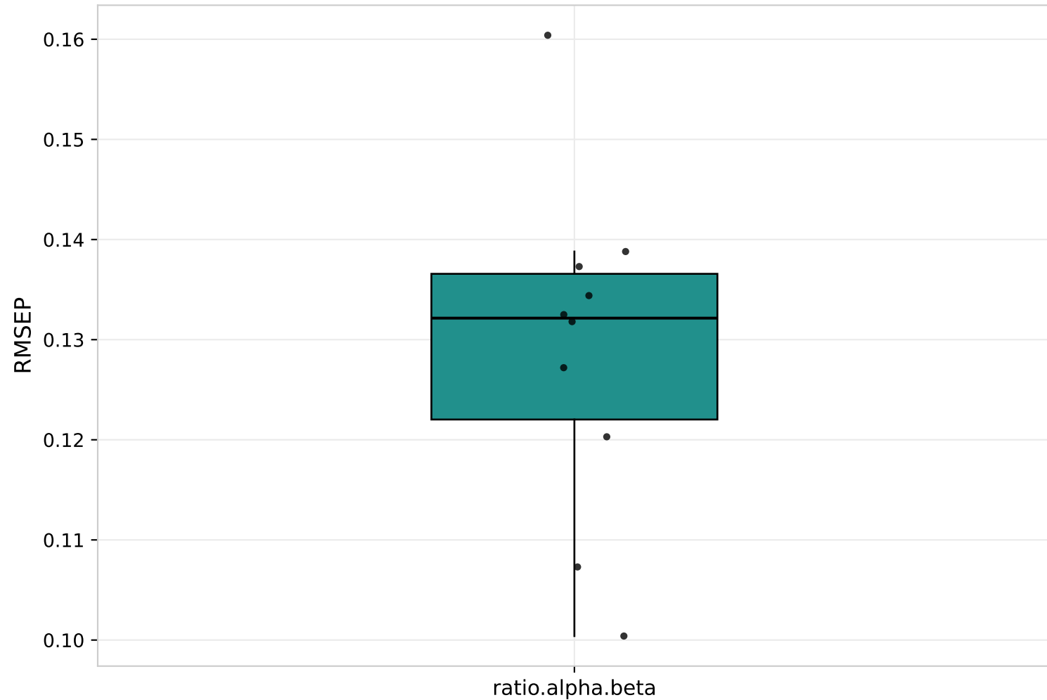
Boxplot des RMSEP obtenus pour ratio.alpha.beta sur les 10 iterations
