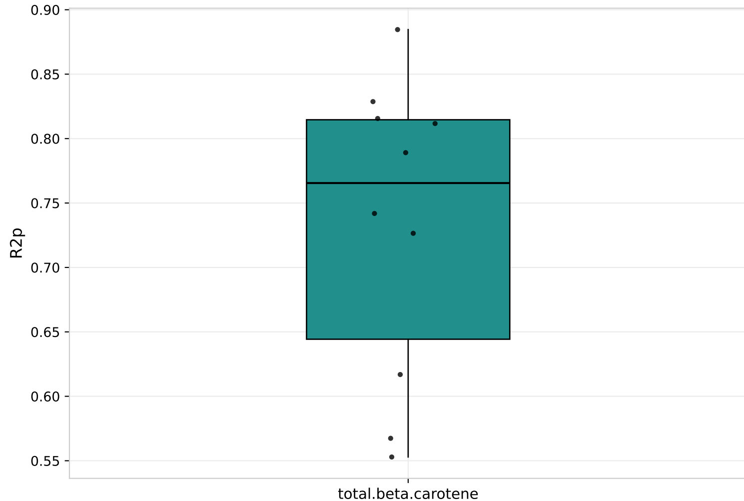
Boxplot des R2p obtenus pour total.beta.carotene sur les 10 iterations
