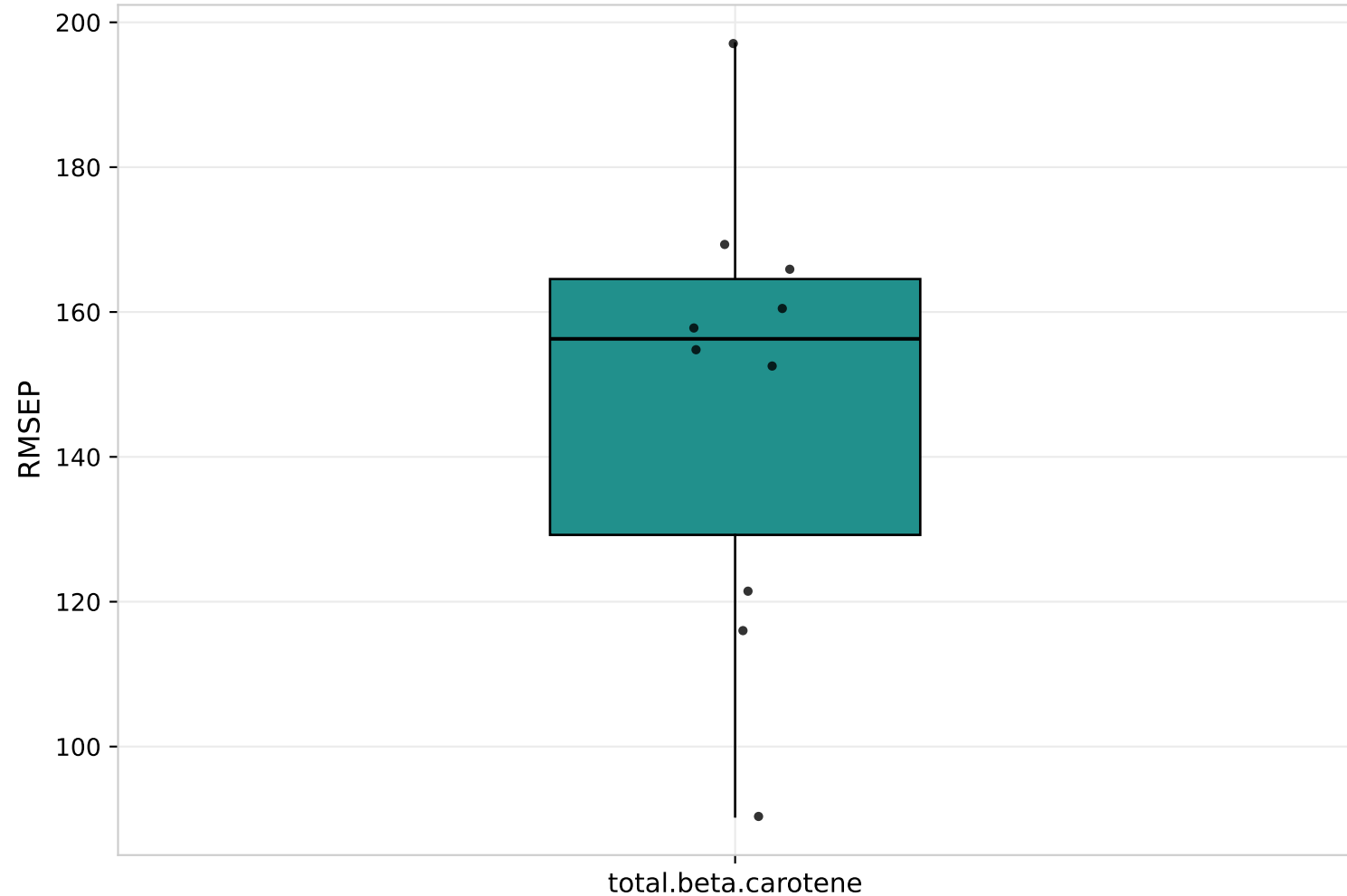
Boxplot des RMSEP obtenus pour total.beta.carotene sur les 10 iterations
