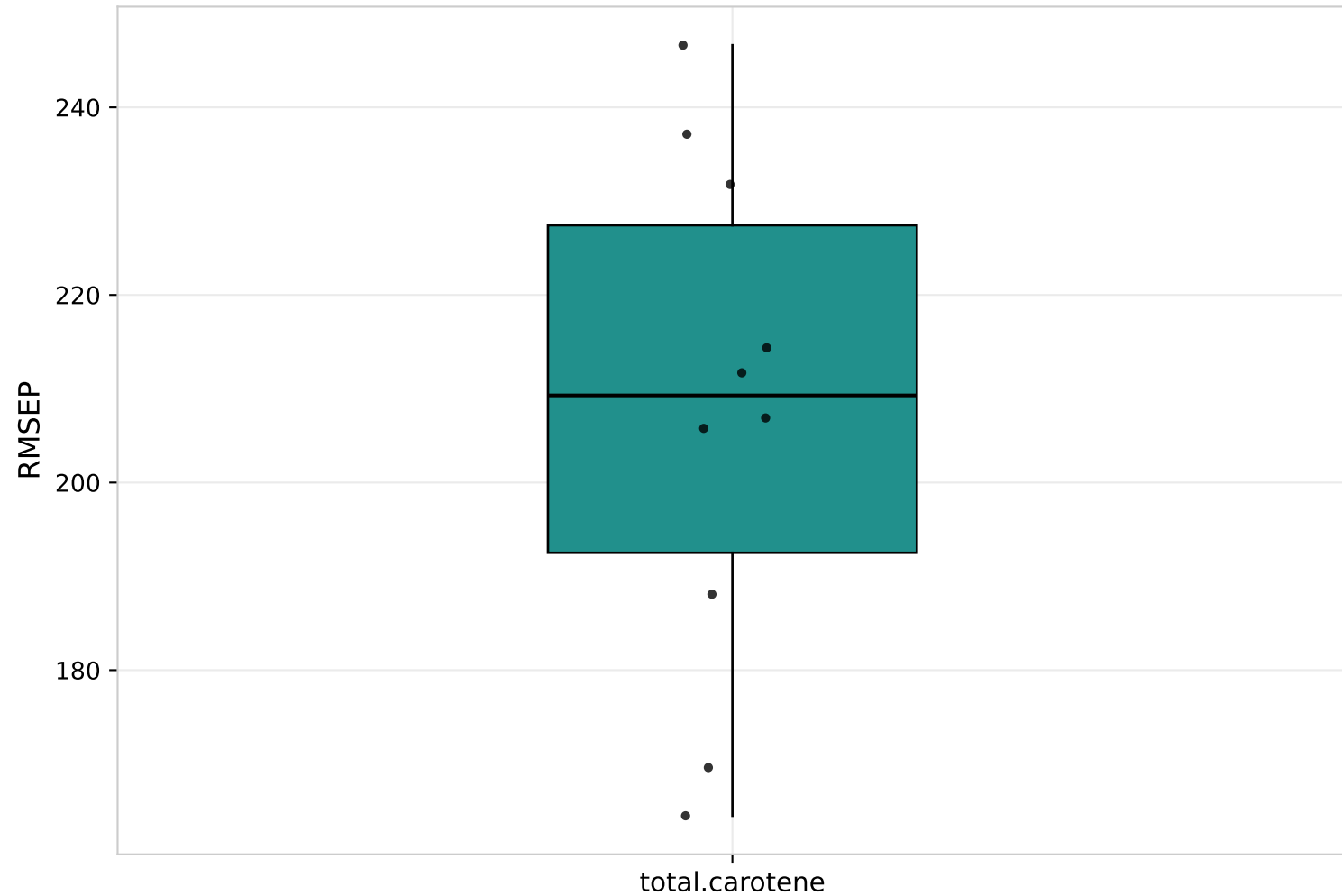
Boxplot des RMSEP obtenus pour total.carotene sur les 10 iterations
