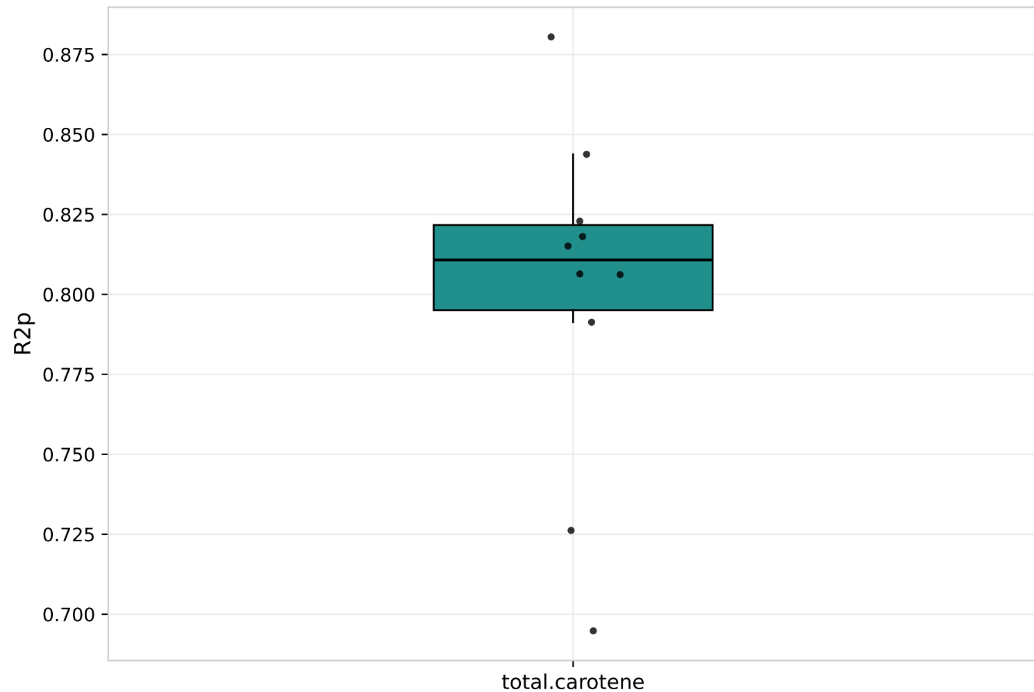
Boxplot des R2p obtenus pour total.carotene sur les 10 iterations
