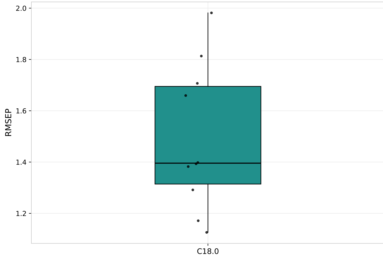
Boxplot des RMSEP obtenus pour C18.0 sur les 10 iterations
