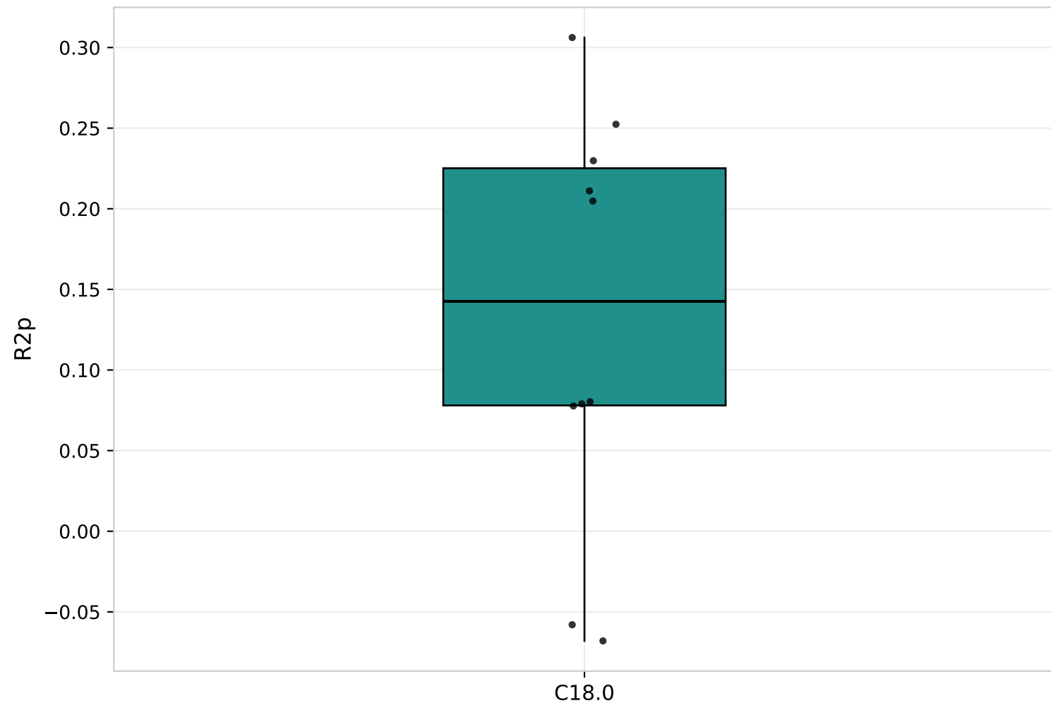
Boxplot des R2p obtenus pour C18.0 sur les 10 iterations
