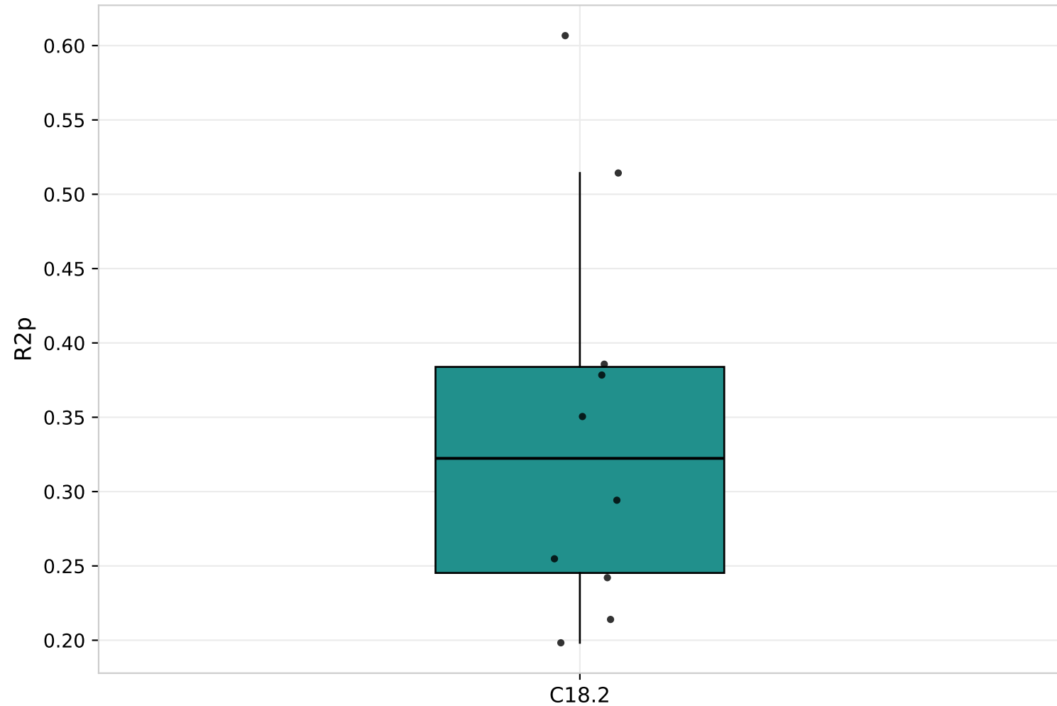
Boxplot des R2p obtenus pour C18.2 sur les 10 iterations
