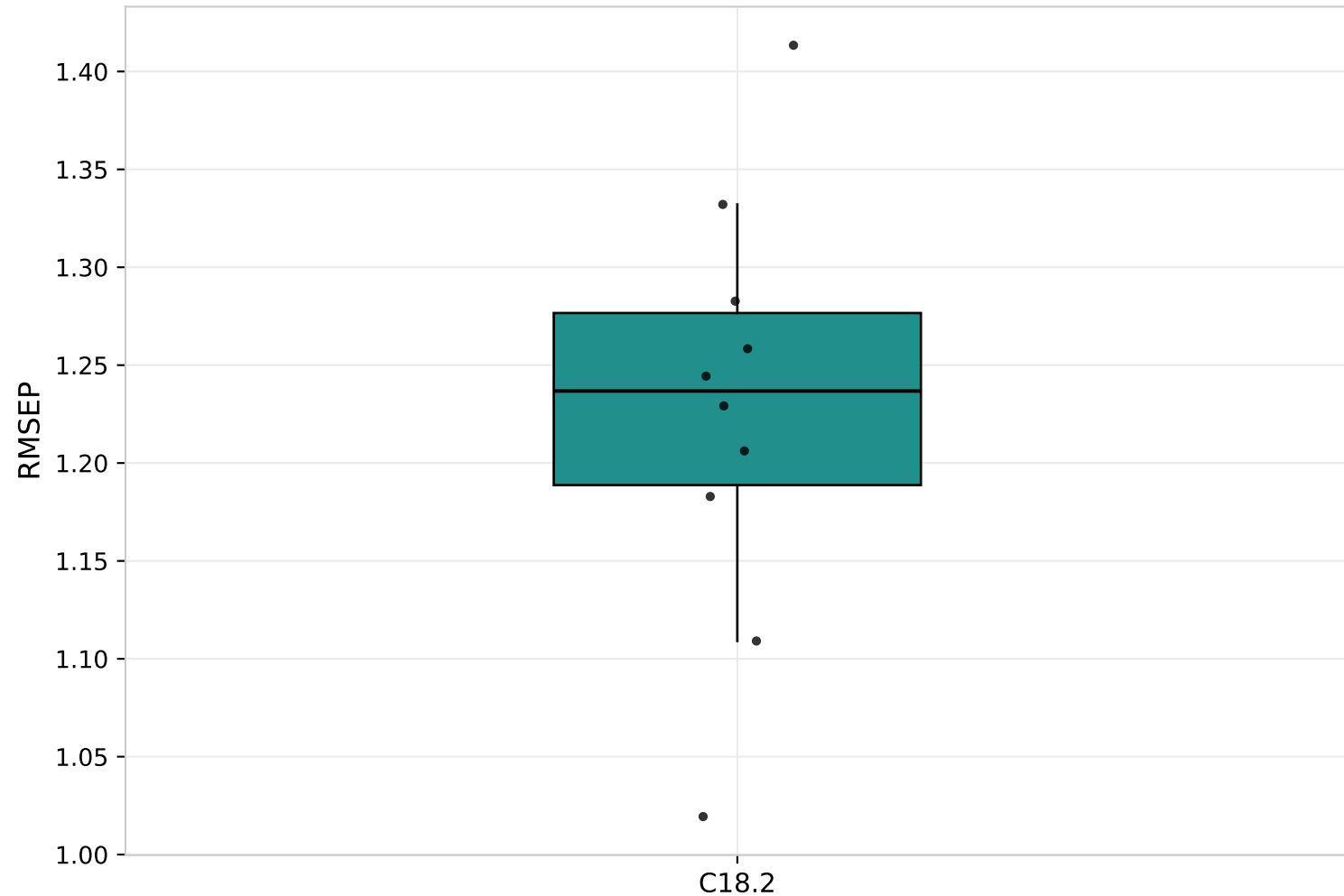
Boxplot des RMSEP obtenus pour C18.2 sur les 10 iterations
