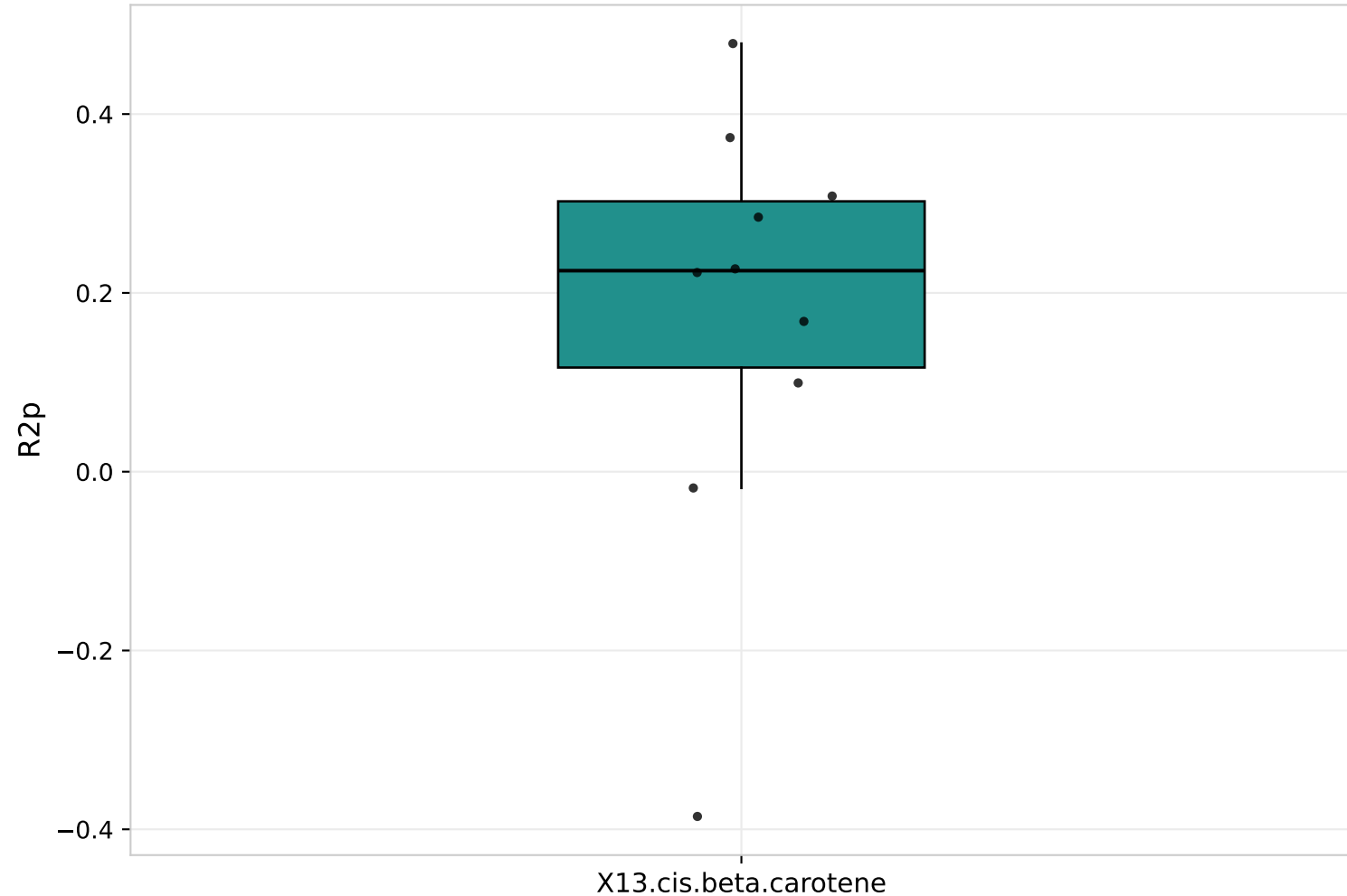
Boxplot des R2p obtenus pour X13.cis.beta.carotene sur les 10 iterations
