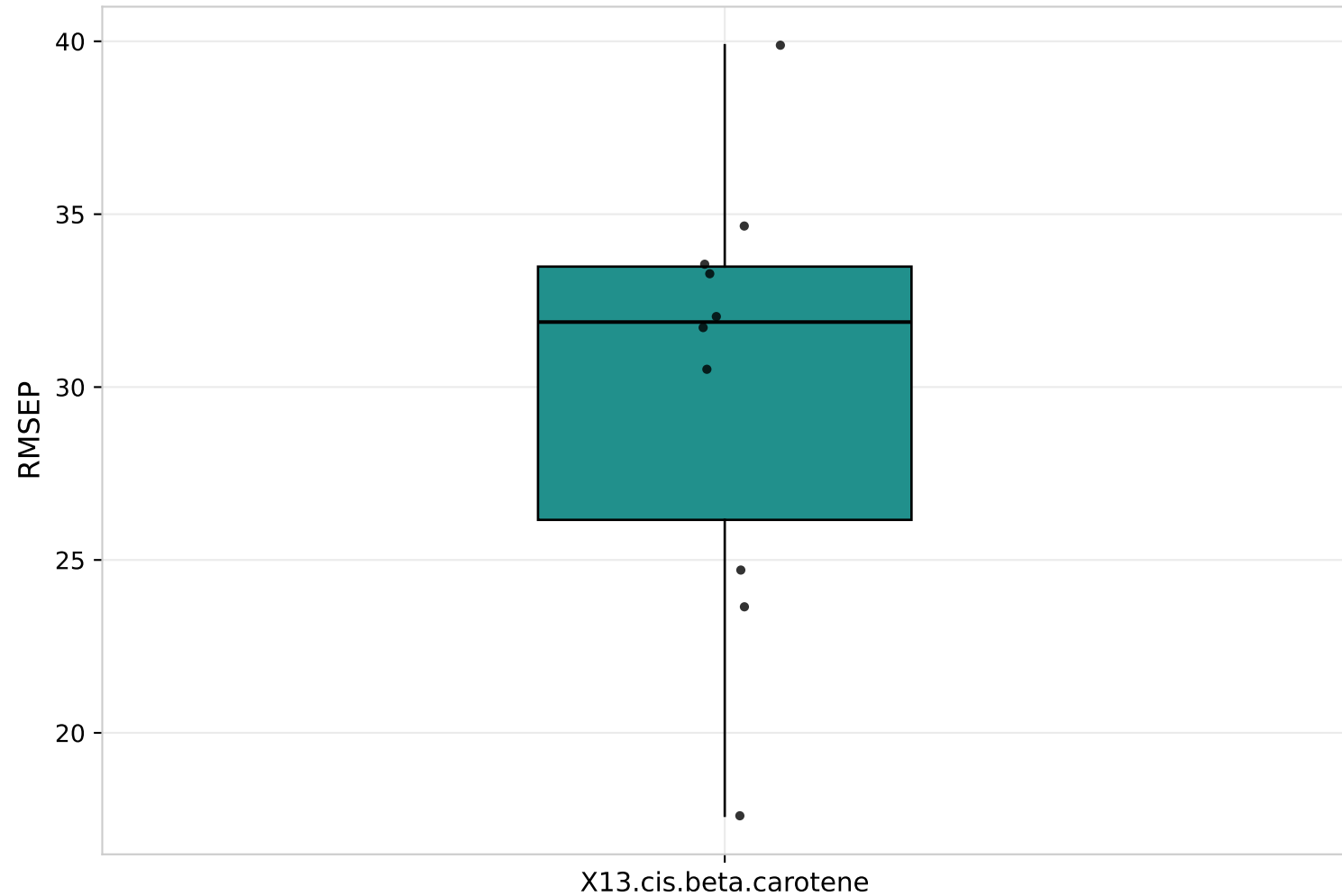
Boxplot des RMSEP obtenus pour X13.cis.beta.carotene sur les 10 iterations
