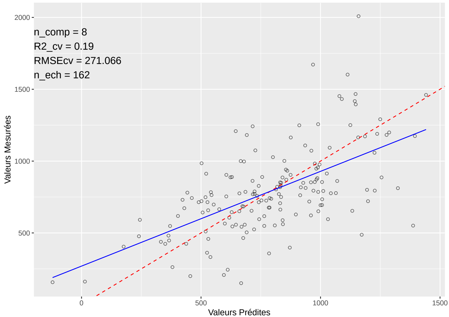
Prédictions vs Mesures : total.toco
