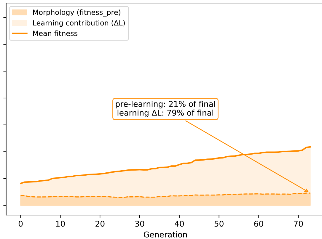
NSGA-II
