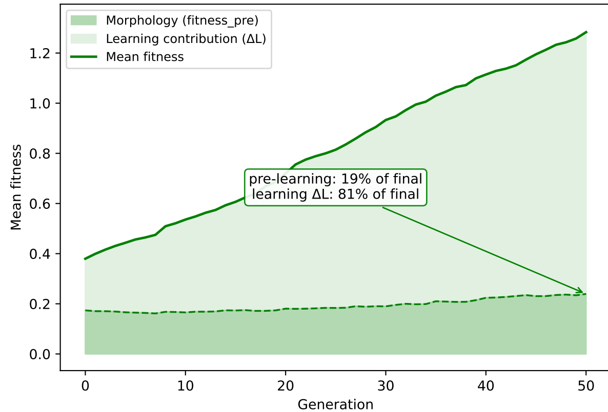
Baseline
