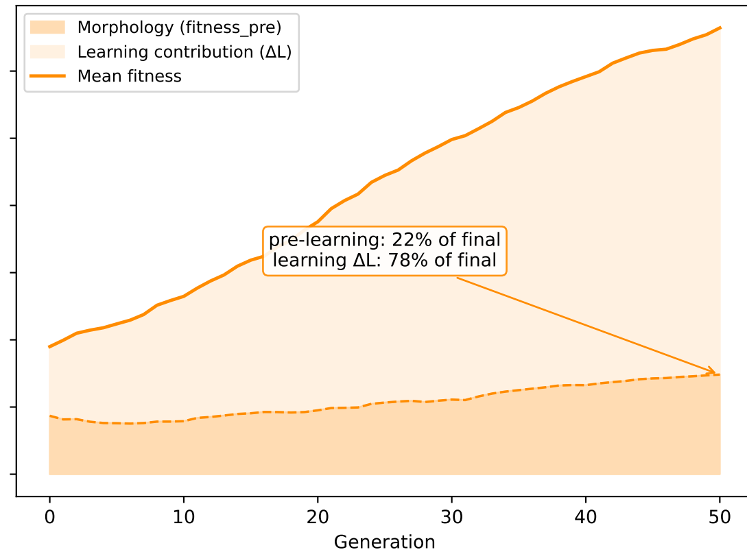
NSGA-II
