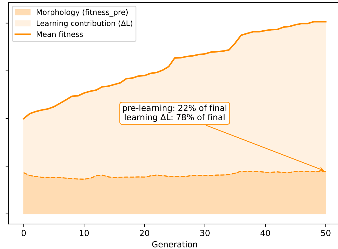
NSGA-II
