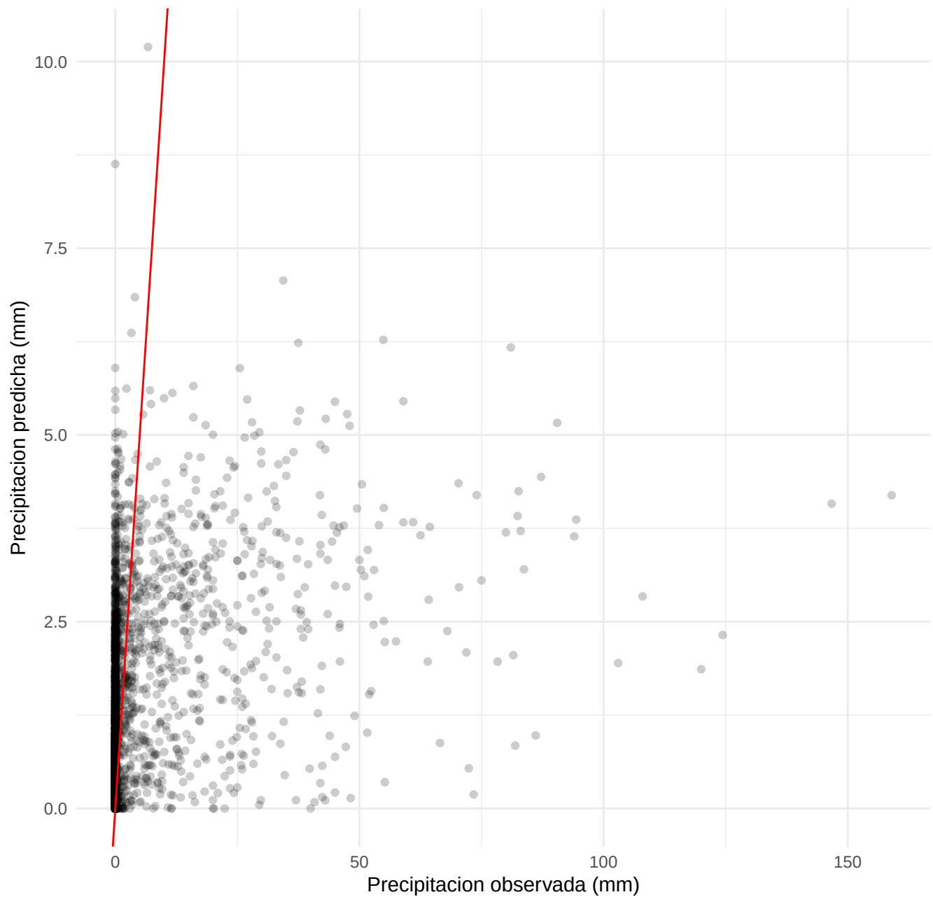
Modelo logaritmico: precipitacion observada y predicha
