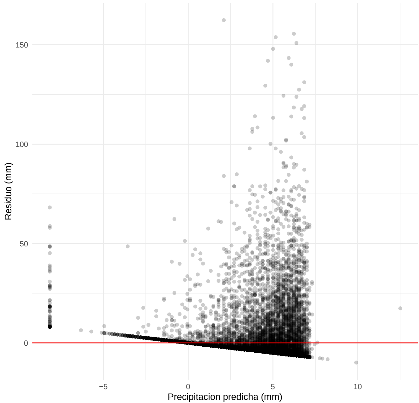
Residuos del modelo simple
