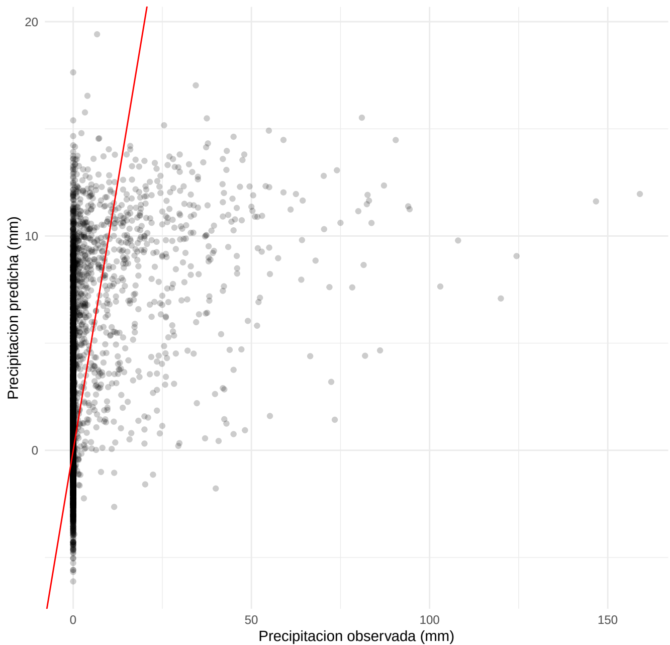
Modelo multiple: precipitacion observada y predicha
