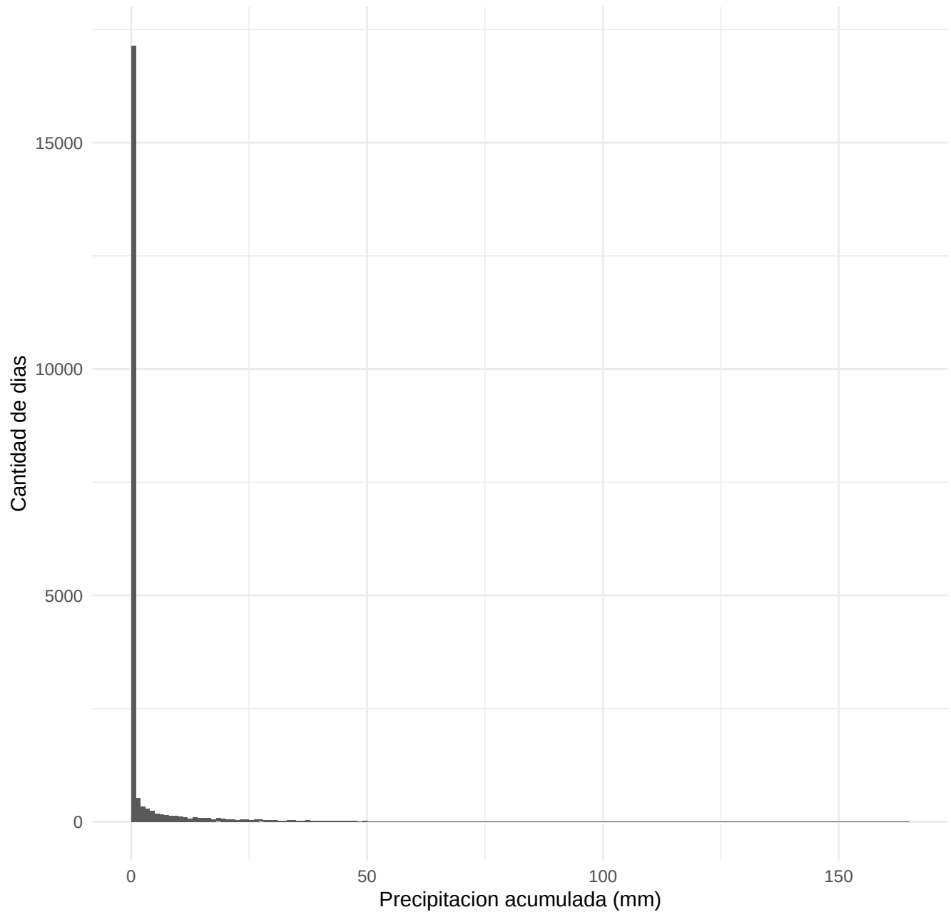
Distribucion de la precipitacion acumulada diaria
