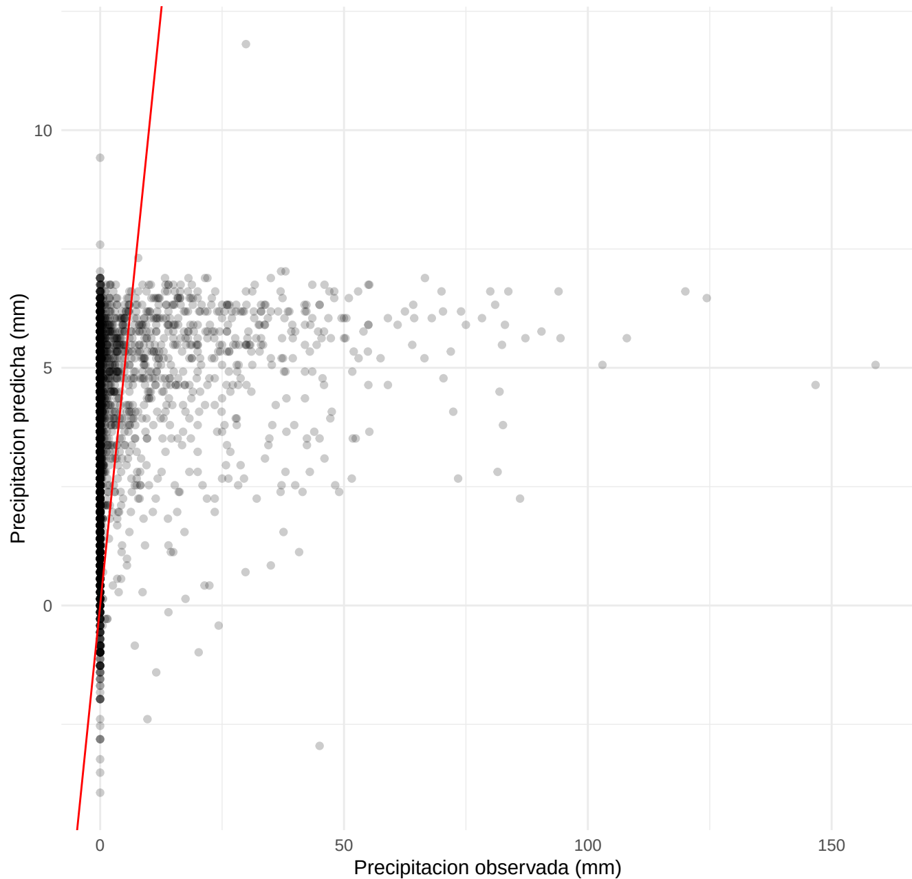
Precipitación observada y predicha: conjunto de evaluacion
