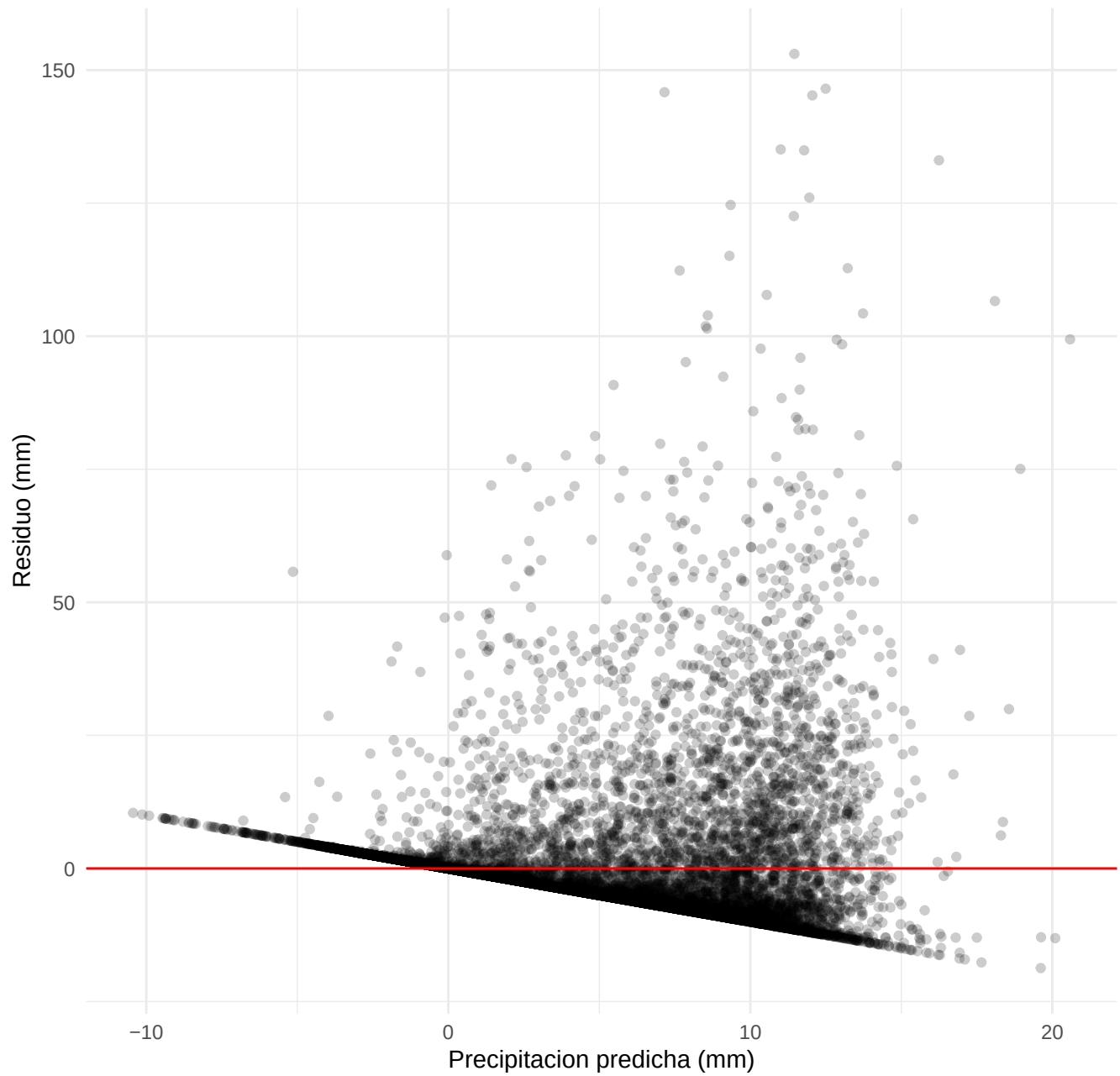
Residuos del modelo multiple
