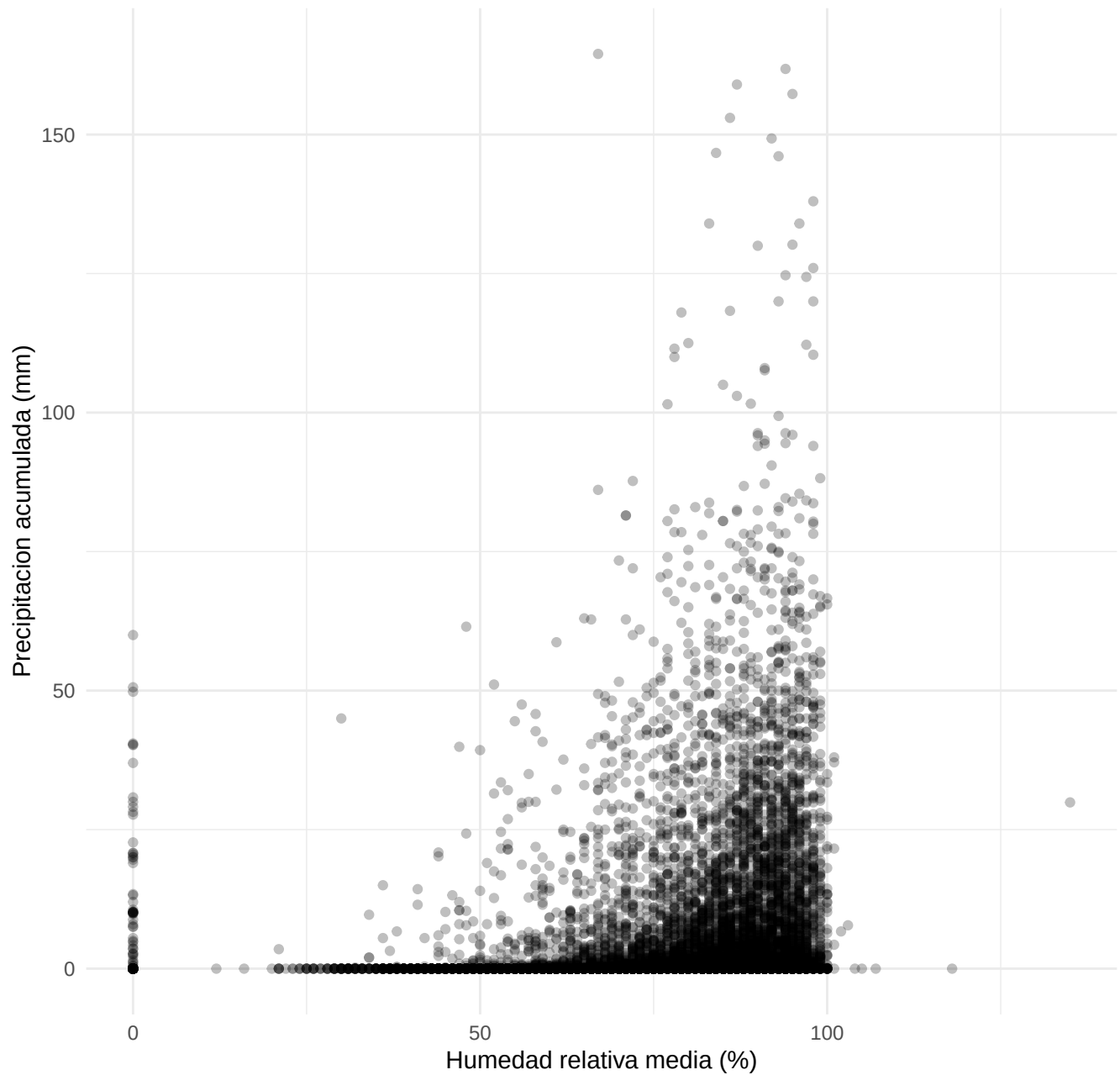
Precipitación acumulada y humedad relativa media
