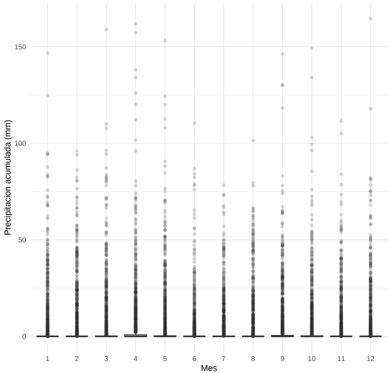
Precipitacion acumulada por mes
