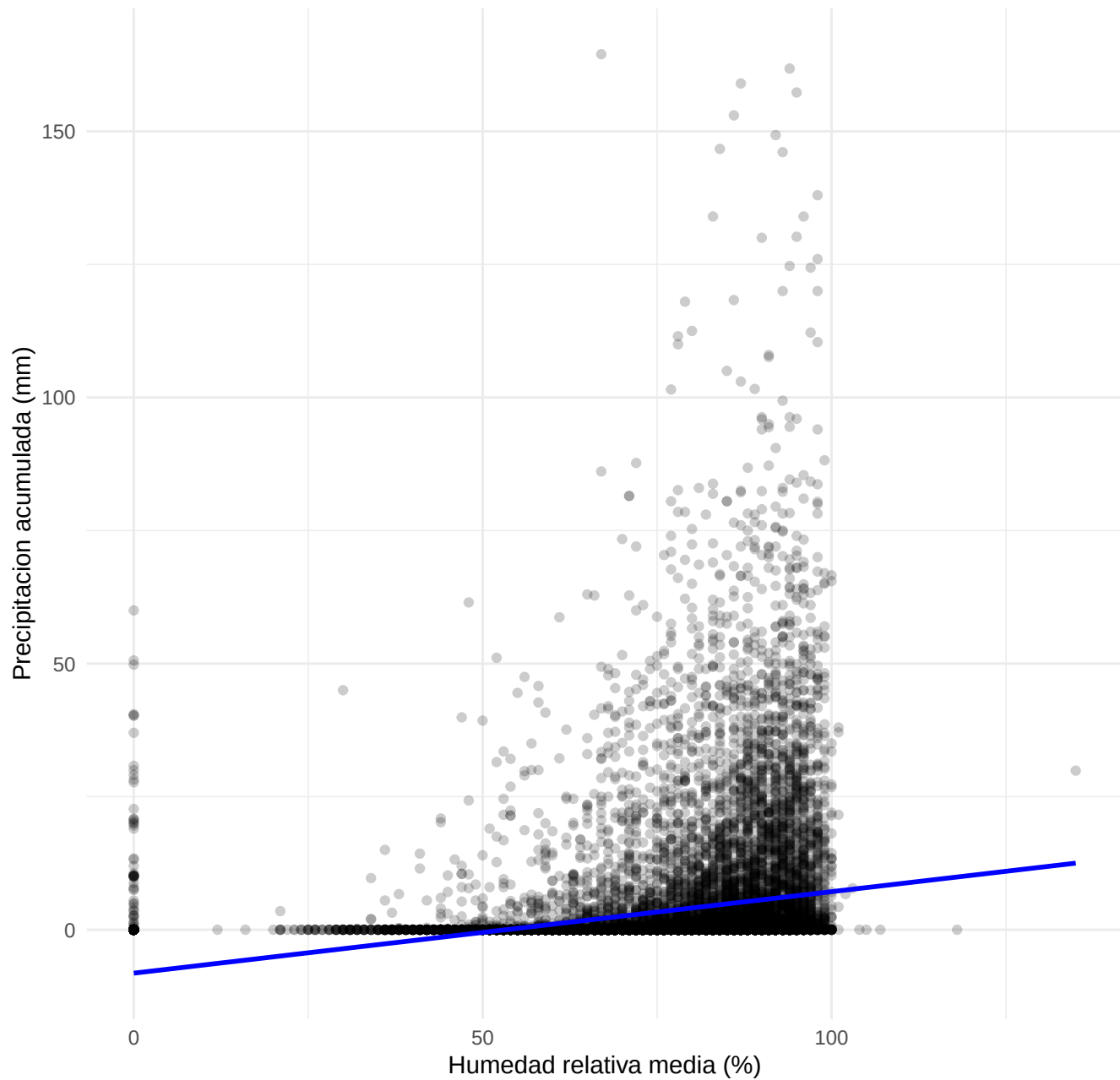
Regresión lineal: precipitación y humedad relativa media
