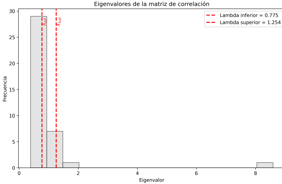
Figura 6.2: Distribución empírica de los valores propios comparada con los límites de Marčenko–Pastur.
