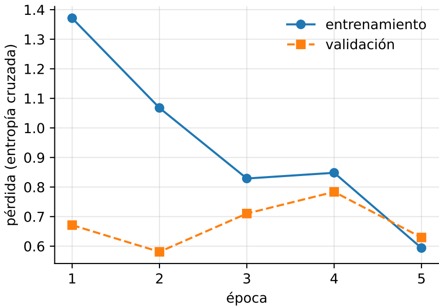
xlm-t_fakedes_s42
