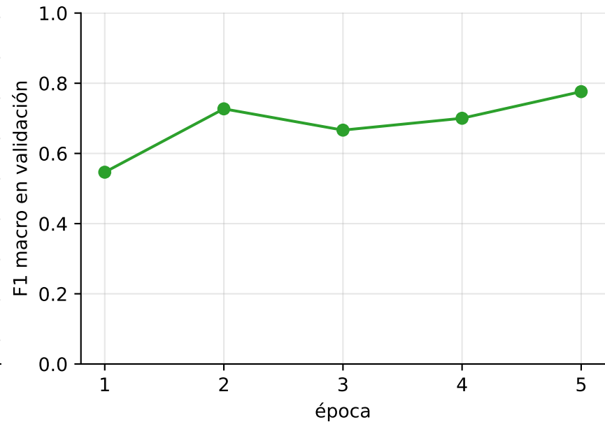
xlm-t_fakedes_s42
