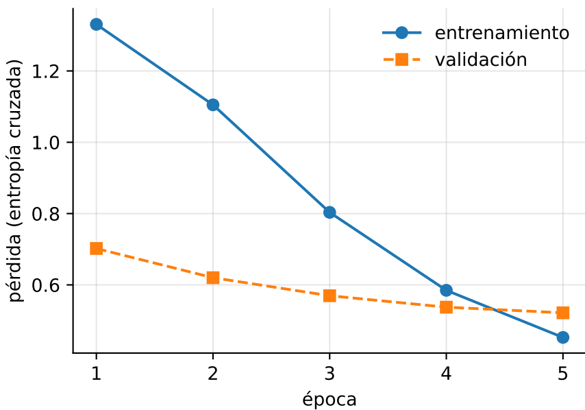
robertuito_fakedes_s42
