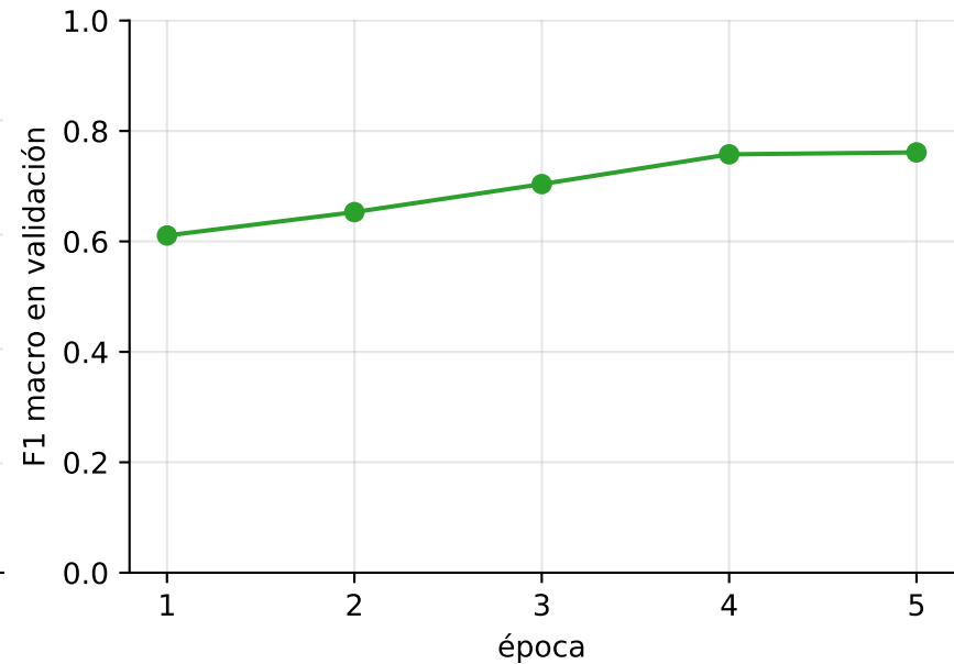
robertuito_fakedes_s42
