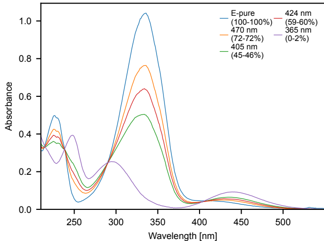
example_data/data_photoswitch-AAP40.xlsx
