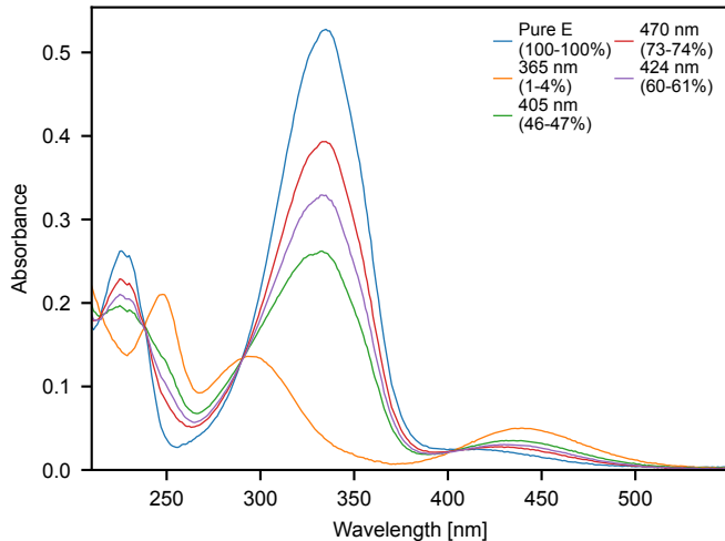
example_data/data_photoswitch-AAP20.xlsx
