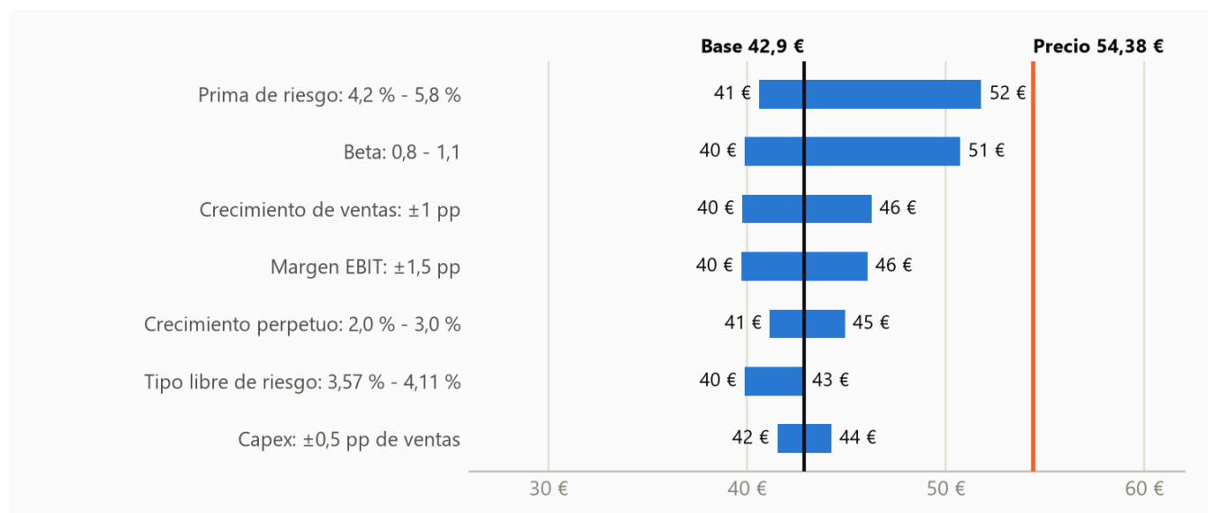
Figura 3. Valor por acción (escenario Base) al cambiar una hipótesis cada vez entre su extremo bajo y alto.
