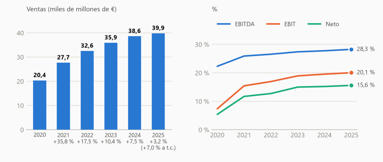
Figura 2. Ventas (miles de millones de €, con su variación anual) y márgenes sobre ventas, ejercicios 2020-2025.
