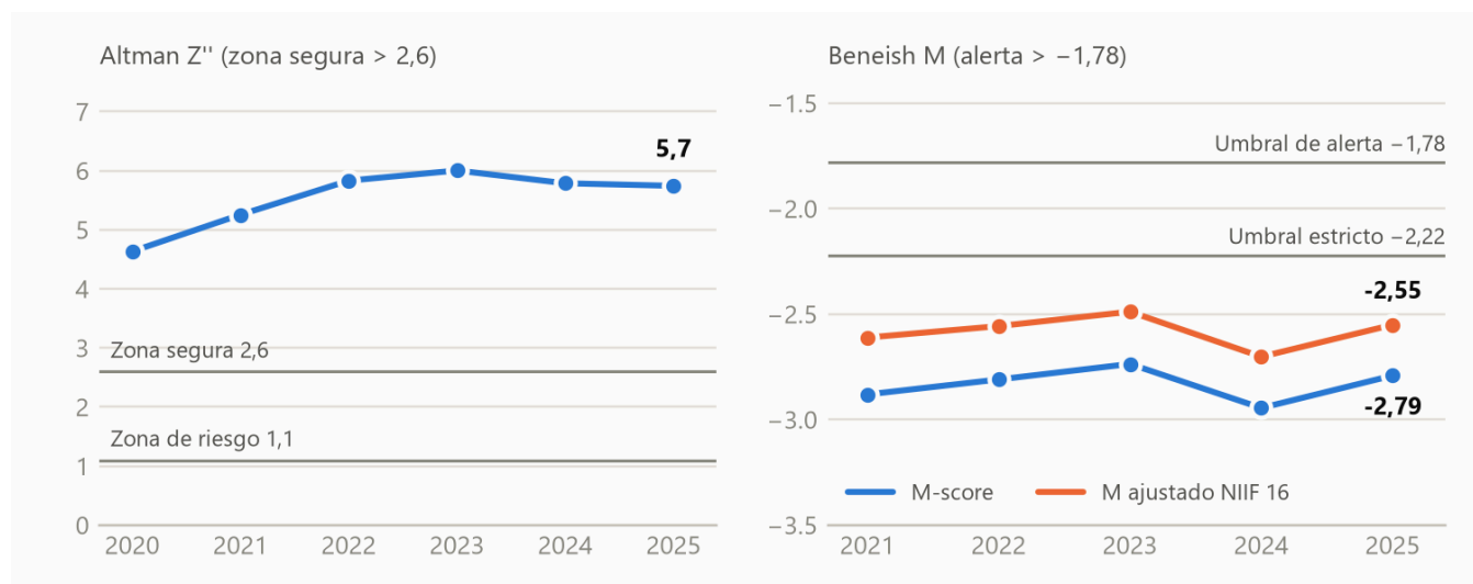
Figura 5. Altman Z'' (izquierda) y Beneish M-score (derecha) de Inditex.
