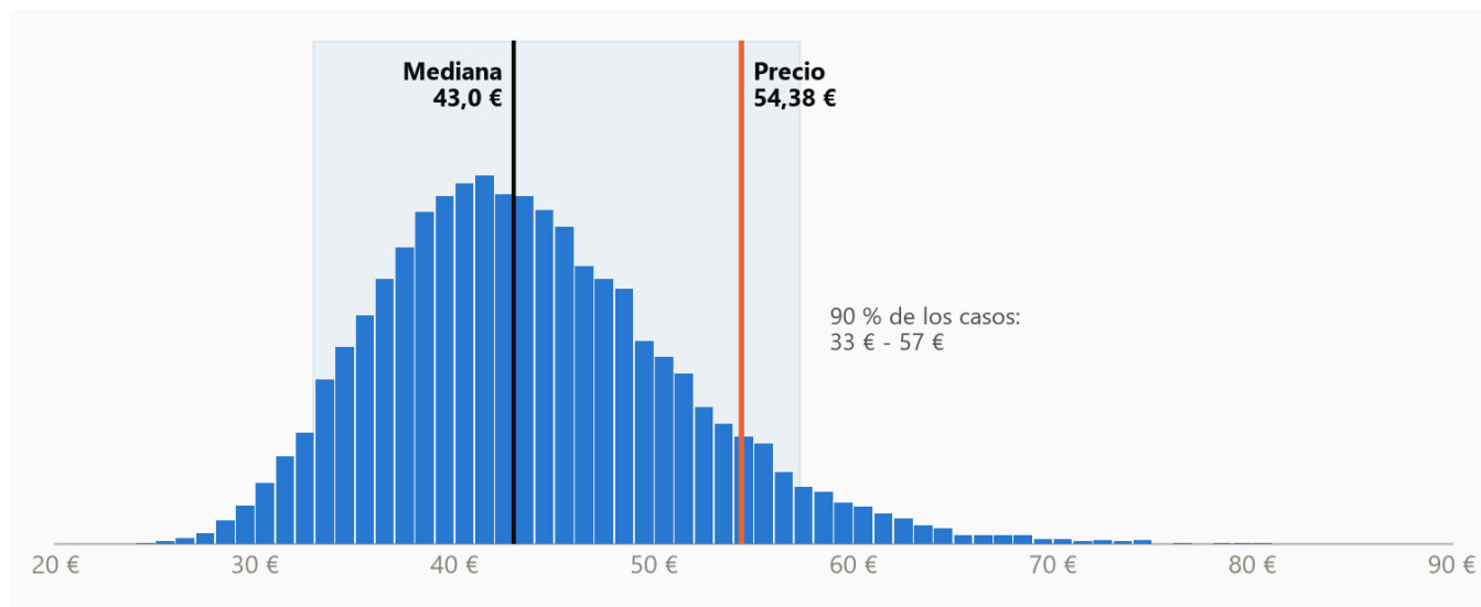
Figura 4. Distribución del valor por acción en 20.000 simulaciones. Banda sombreada: 90 % de los casos.
