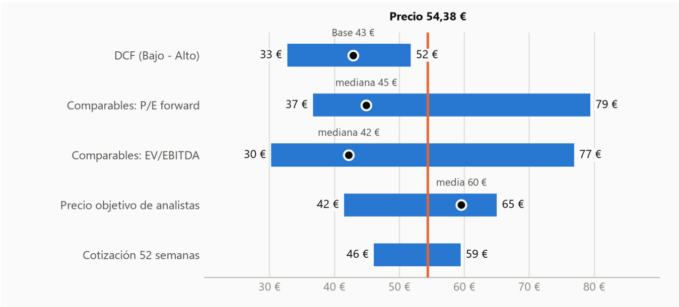
Figura 1. Valor por acción según cada método frente al precio de mercado (campo de fútbol). Punto = valor central.
