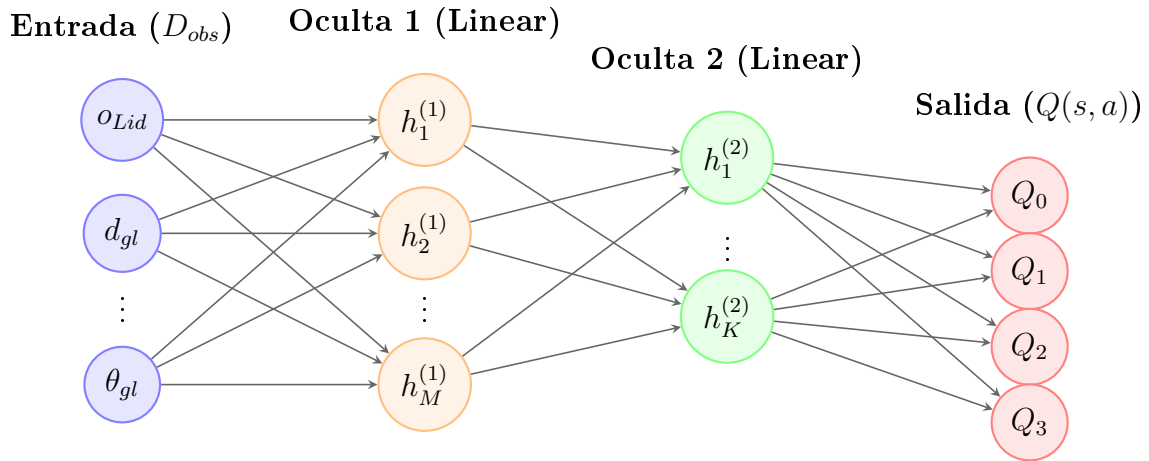
Figura 3.1: Diagrama visual de conexiones de la arquitectura de la red SimpleQNetwork de control adaptada a los espacios de acción discretos del AGV ( |A| = 3 para GridRobot y |A| = 4 para GridRobotNotTurning ).
