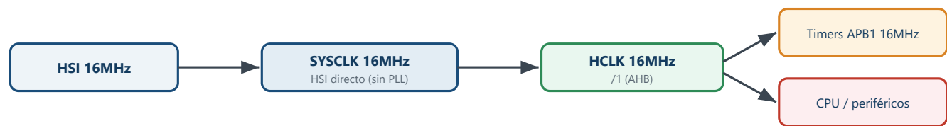
Figura 2 — Cadena de reloj (HSI directo, sin PLL). Los timers APB1 quedan a 16 MHz.
