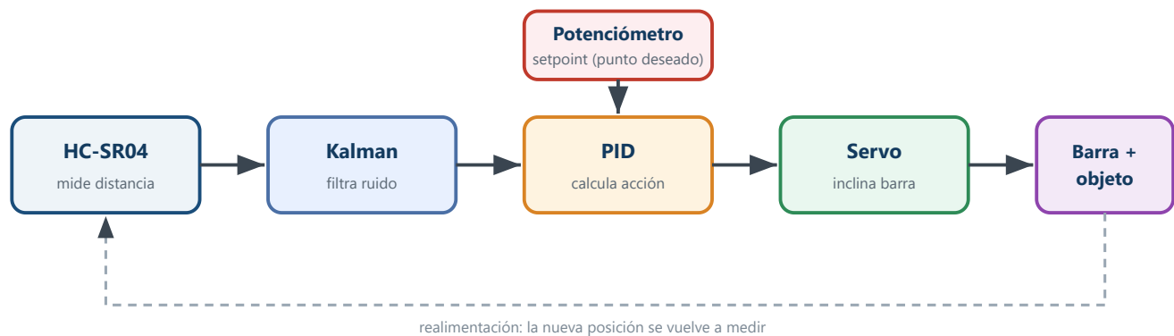
Figura 1 — Lazo de control cerrado del ball-and-beam.
