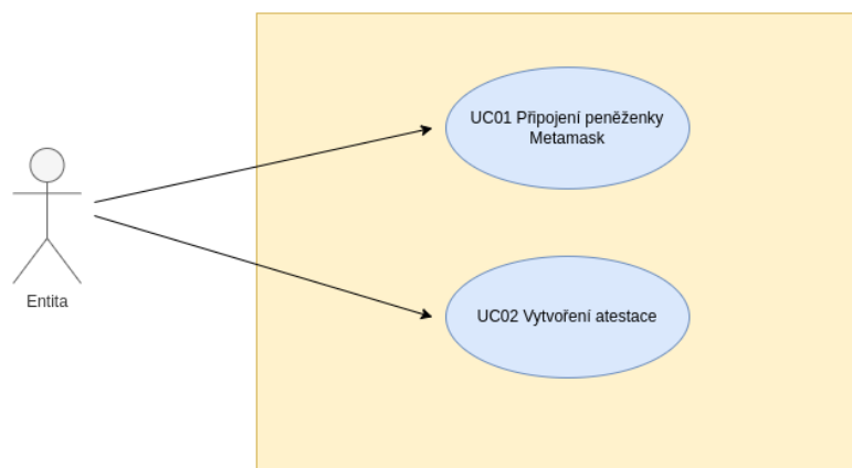
Obr. 4.1 Diagram případu použití Entita
