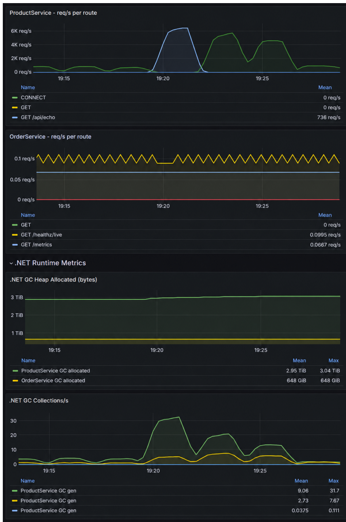
Rysunek 6.2: Pulpit Grafany – liczba żądań w podziale na trasy oraz metryki środowiska uruchomieniowego .NET: wolumen alokacji i częstość odświeżania pamięci
