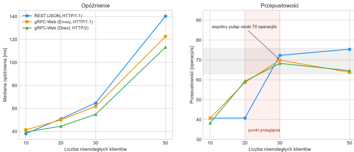
Rysunek 8.6: Opóźnienie i przepustowość względem liczby równoległych klientów; szary pas oznacza wspólny pułap przepustowości, a różowy położenie punktu przegięcia
