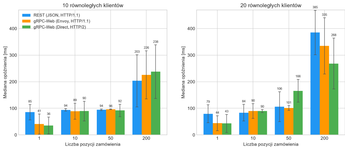
Rysunek 9.4: Mediana opóźnienia w scenariuszach Orders względem liczby pozycji zamówienia; słupki błędów odpowiadają 95% przedziałowi ufności wartości centralnej
