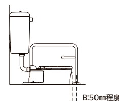
B:便器先端から手すり
