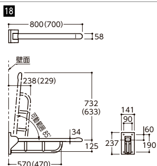
図面はEWC731、( )寸法はEWC730の場合
