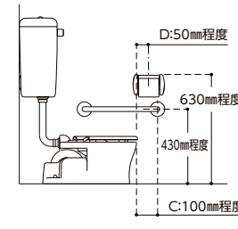
C:便器先端から手すり D:便器先端から紙巻器
