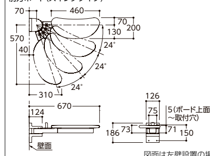
図面は左壁設置の場合
