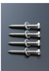
コーチねじ T110D16 希望小売価格 ¥850 コーチねじ(φ6×50): 4本 座金:4個 T110D23 希望小売価格 ¥850 コーチねじ(φ6×30): 4本 座金:4個 T110D55 希望小売価格 ¥2,100 コーチねじ(φ6×50): 9本 座金:9個
