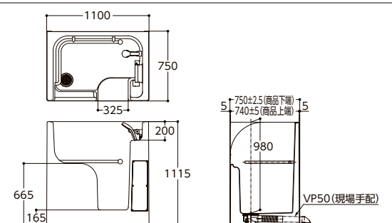
コンフォートウエーブクリックシャワー
