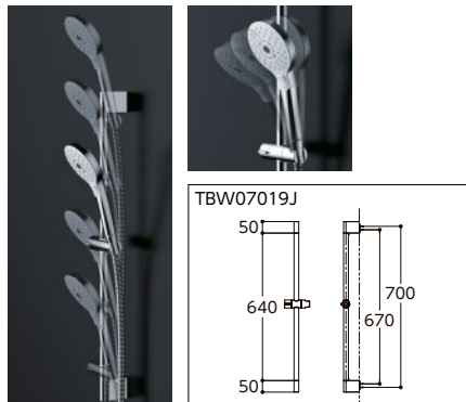
TBW07019J スライドバー
