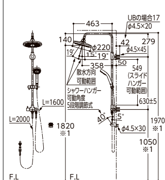
シャワーバー(水栓なしタイプ) TBW04004J1
