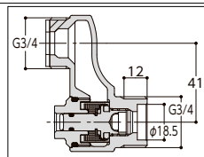
取り替え脚接続部
