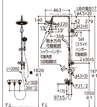
シャワーバー TBW04401J1
