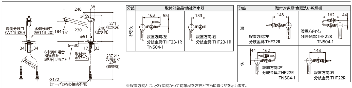
浄水器(水分岐/右設置)とのセット例
