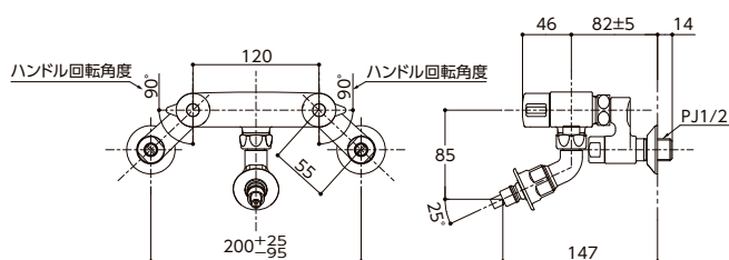
洗濯機用壁付2ハンドル混合水栓 (緊急止水) TW21R
