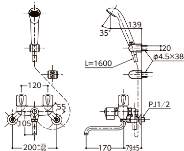
壁付2ハンドル混合水栓 TMS20C
