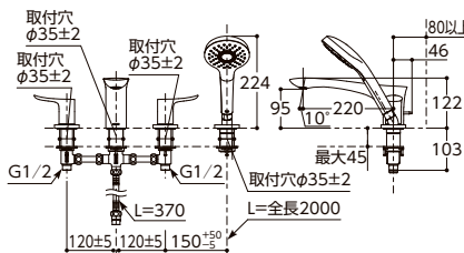
台付2ハンドル混合水栓 TBG01202JA
