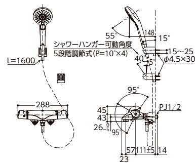
ニューウェーブシリーズ 壁付サーモスタット混合水栓 TMNW40B型
