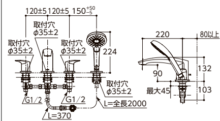
台付2ハンドル混合水栓 TBG09202J
