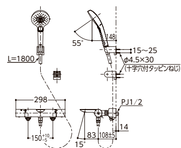
壁付サーモスタット混合水栓 TBV01S06JA・07JA・08JA・12J
