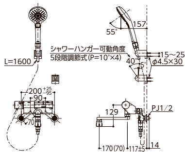
タッチスイッチ 壁付サーモスタット混合水栓 TMN40T型・ST型
