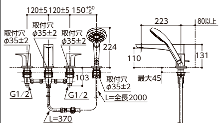
台付2ハンドル混合水栓 TBG07203J
