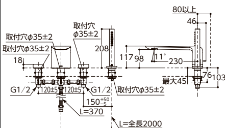
台付2ハンドル混合水栓 ZLシリーズ TBP02202JA
