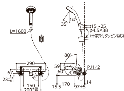
GGシリーズ 壁付サーモスタット混合水栓 TBV03414J1・15J1・16J・17J・52J・56J
