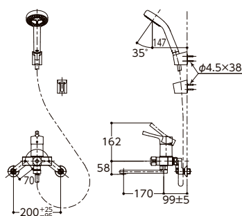
GGシリーズ 壁付シングル混合水栓 TBV03301J1
