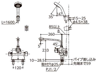
定量止水式 台付サーモスタット水栓 TMJ48Y1
