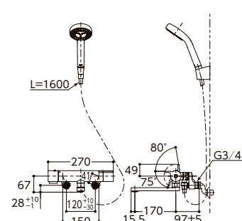
GGシリーズ 壁付サーモスタット混合水栓(取り替え用) TBV03422J1
