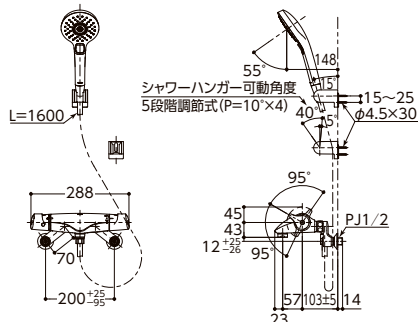
ニューウェーブシリーズ 壁付サーモスタット混合水栓 TMNW40A型
