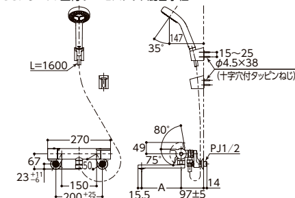
GGシリーズ 壁付サーモスタット混合水栓
