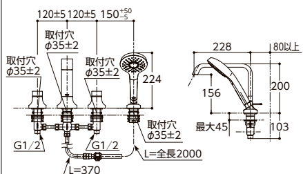
台付2ハンドル混合水栓 TBG08203J
