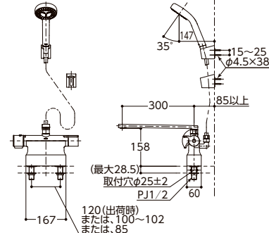
GGシリーズ 台付サーモスタット混合水栓(取り替え用) TBV03423J1・24J1・53J
