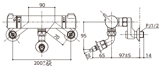
洗濯機用壁付2ハンドル混合水栓 (緊急止水) TW21R
