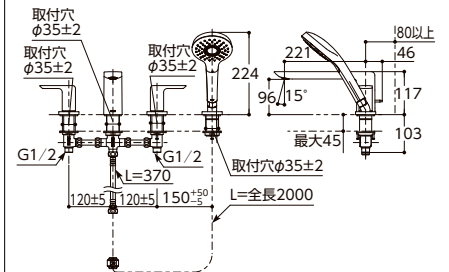
台付2ハンドル混合水栓 TBG02202JA
