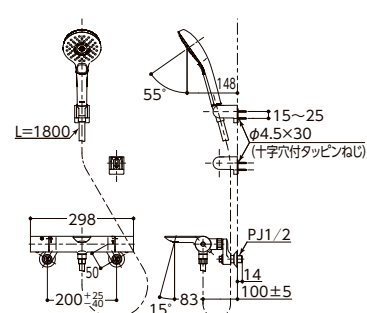
壁付サーモスタット混合水栓 TBV01S01JA・02JA・03JA・11J
