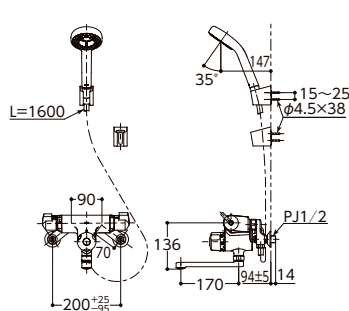
定量止水式 壁付サーモスタット混合水栓 TMF47Y1
