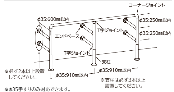
エンドベース >>> 532ページ
