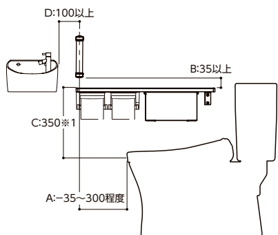
YHBS203FBRの場合
