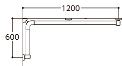
セット図
