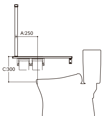
YHBS203FRの場合
