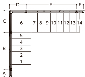
セット図
