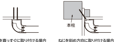
ねじを真っすぐに取り付ける場合 ねじを斜め方向に取り付ける場合
