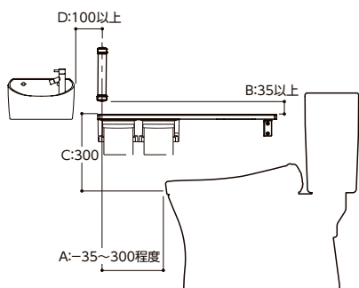
YHBS203FRの場合
