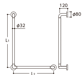
TS134GLMY8#NW1 希望小売価格 ¥32,200
