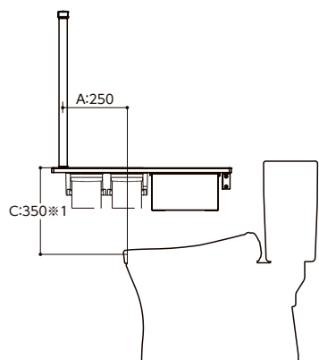
YHB63FBRの場合
