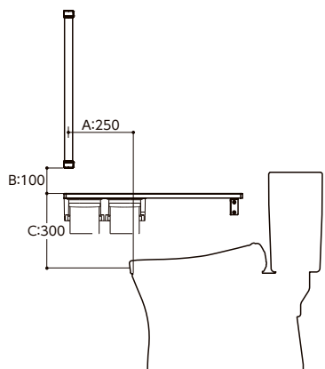
YHB63FRの場合
