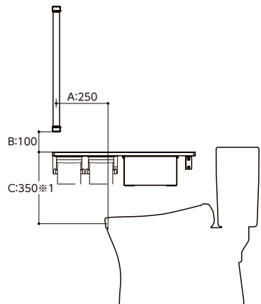
YHB63NBR、YHBS603FBRの場合
