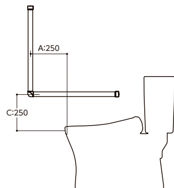
YHB603Lの場合
