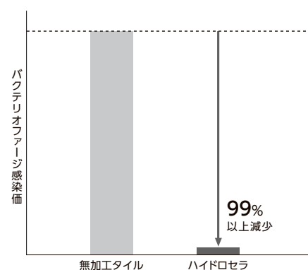
抗ウイルス効果/バクテリオファージ感染価比較※2
