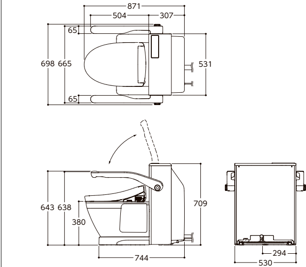
ベッドサイド水洗トイレ
