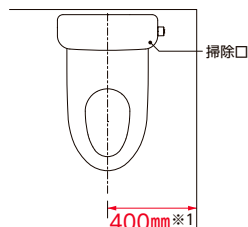
パブリックコンパクト便器・タンク式 (CS597BCS・BLCS・BMCS・BMLCS・ BPC・BPLC系)
