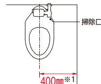
パブリックコンパクト便器・フラッシュバルブ式 (CS494J・LJ・MJ・MLJ系)
