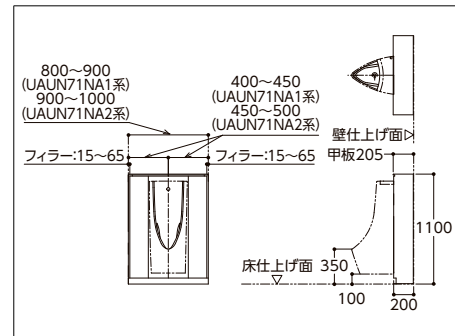
UFS900系と点検口付ライニング(UAUN7系)とのセット例
