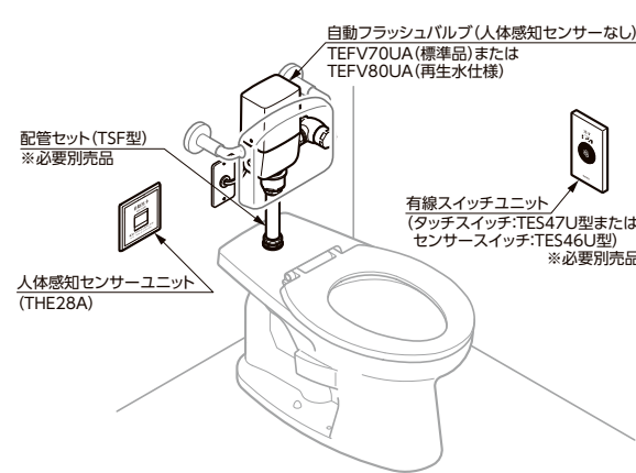
人体感知センサーユニットをセットする場合
