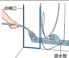
UFS900系と点検口付ライニング(UAUN7系)とのセット例
