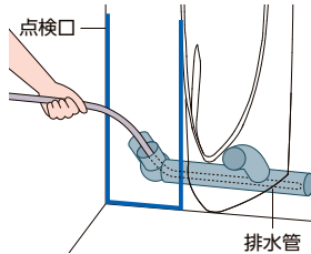
UFS900系と点検口付ライニング(UAUN7系)とのセット例
