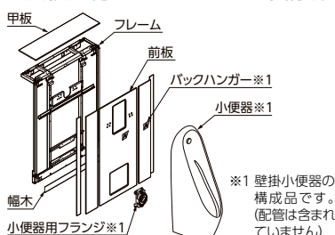
UFS900系と点検口付ライニング(UAUN7系)とのセット例
