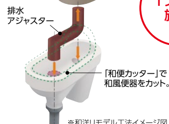
※和洋リモデル工法イメージ図
