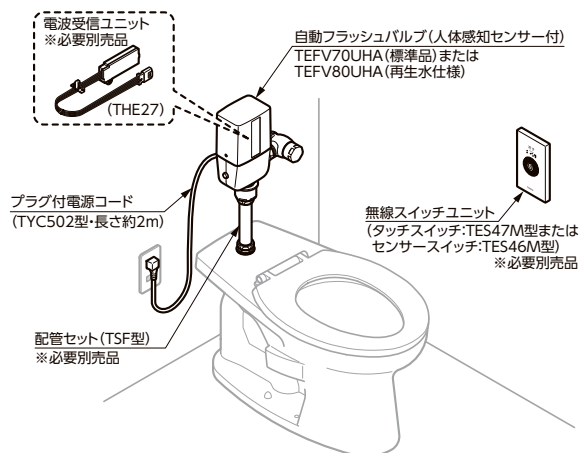
便ふたなしの便座・ウォシュレットに設置する場合
