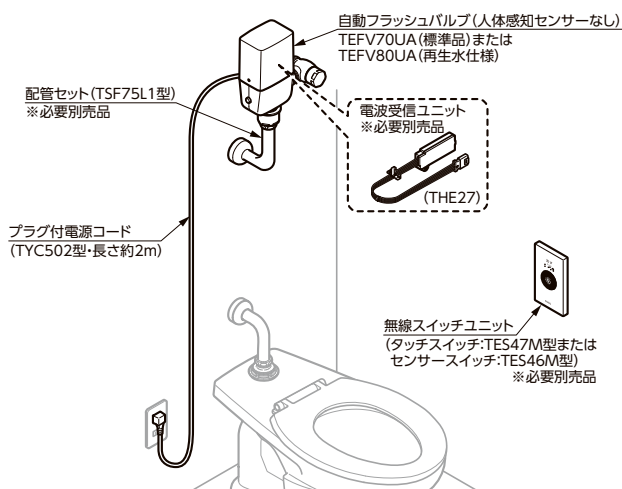
リモコンフラッシュバルブ(壁給水壁排水)からの交換の場合
