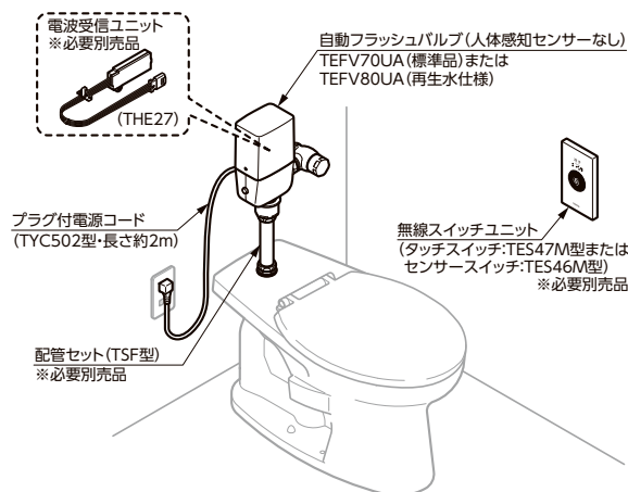
便ふたありの便座・ウォシュレットに設置する場合
