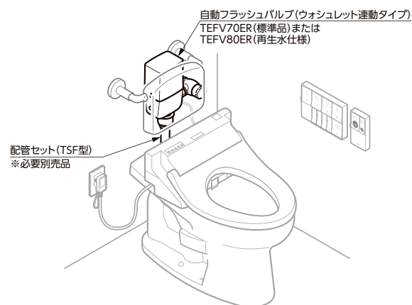
ウォシュレット連動タイプをセットする場合
