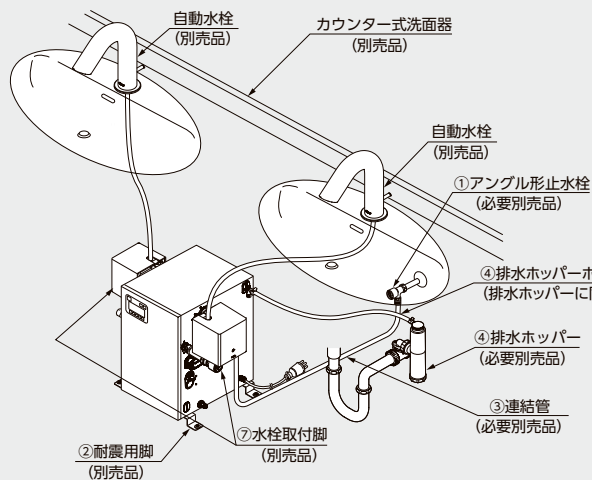
品番 REW-D 自動水栓(単水栓)
