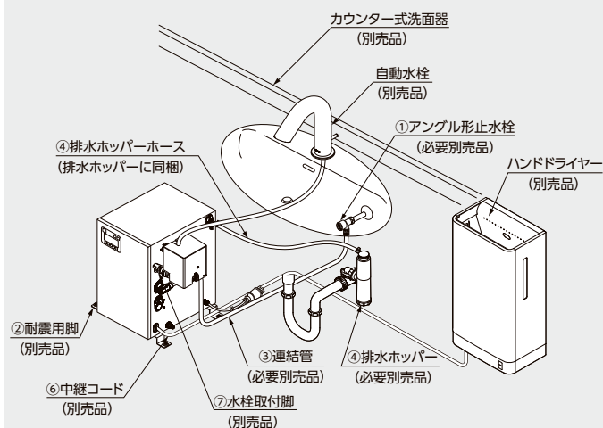
品番 REW-B ハンドドライヤーと電気温水器(機器連動した場合)
