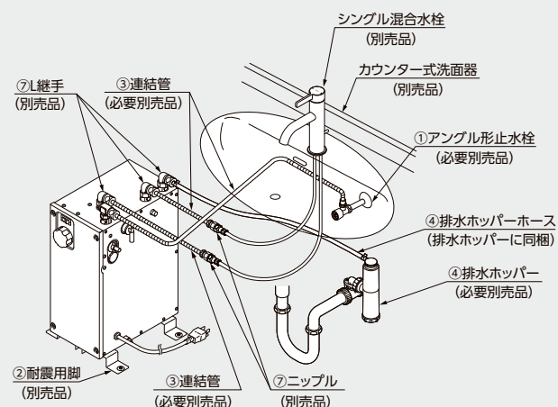
品番 REW06-E シングル混合水栓
