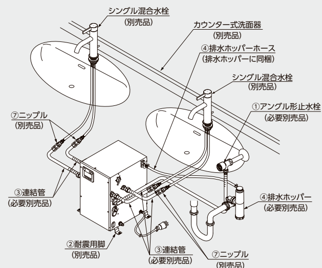
品番 REW-B/REW-D シングル混合水栓
