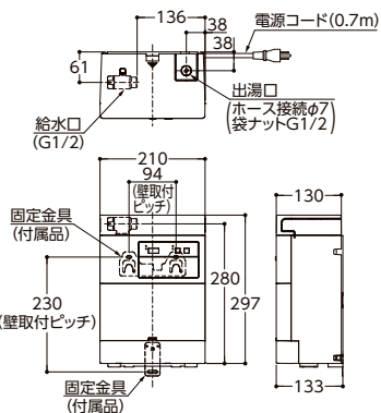
品番 RECK03/REAH03-REAK03/REAL03
