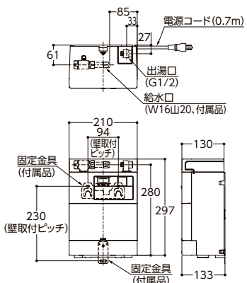
品番 REBH03
