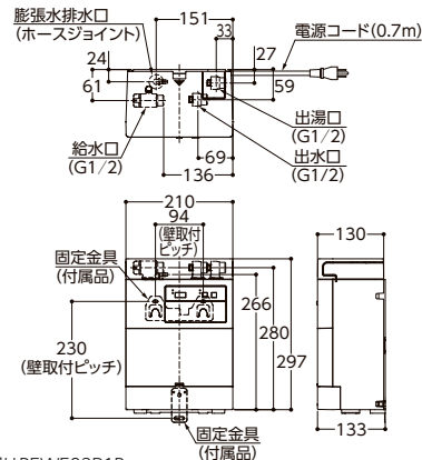
品番 REWF03
