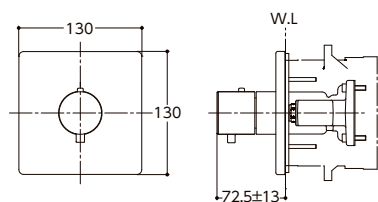
壁付サーモスタット混合水栓 (埋込式) サーモ TBV02401J
