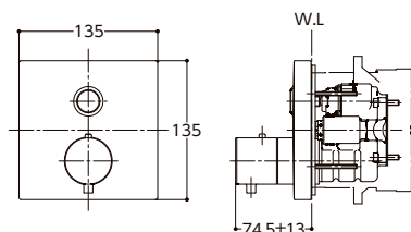
壁付サーモスタット混合水栓 (埋込式) サーモタッチ止水付き TBV02405J
