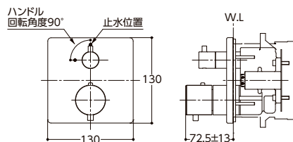
壁付サーモスタット混合水栓 (埋込式) サーモ止水付き TBV02403J
