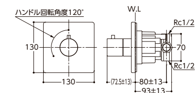
切り替えバルブ (埋込式) 切替2way止水なし TBV02103J
