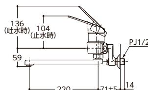
壁付シングル混合水栓 T330DR
