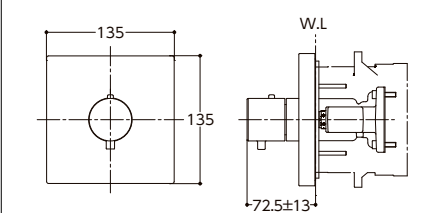
壁付サーモスタット混合水栓 (埋込式) サーモ[タッチ切替3way専用] TBV02402J
