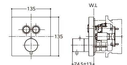
壁付サーモスタット混合水栓 (埋込式) サーモタッチ切替2way止水付き TBV02406J
