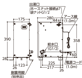
品番 REAH06-REAK06
