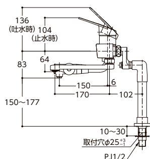
台付シングル混合水栓(飲料熱湯用) T336DR
