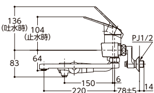
壁付シングル混合水栓(飲料熱湯用) T335DR
