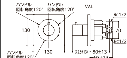
切り替えバルブ (埋込式) 切替3way止水なし TBV02104J
