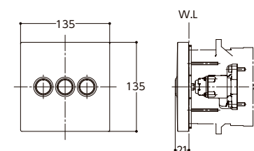
切り替えバルブ (埋込式) タッチ切替3way止水付き TBV02105J
