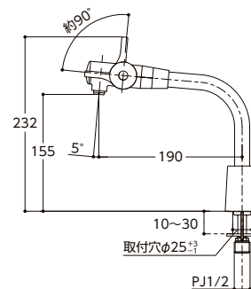
立水栓(飲料熱湯用) T76D
