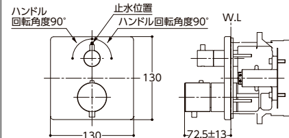
壁付サーモスタット混合水栓 (埋込式) サーモ切替2way止水付き TBV02404J
