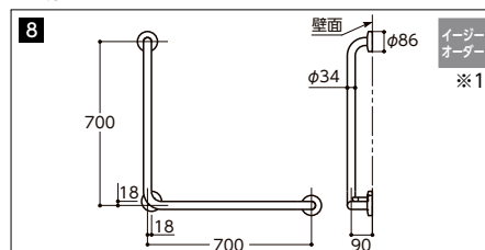
T112CL9#NW1 希望小売価格 ¥46,200 長さ:700×700mm 握り径:φ34mm 抗菌
