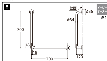
T112CL10#NW1 希望小売価格 ¥52,900 長さ:700×700mm 握り径:φ34mm 抗菌
