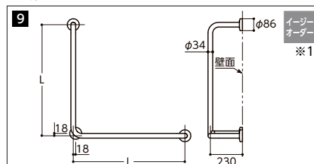
T112CL11#NW1 希望小売価格 ¥58,400 長さ:800×800mm 握り径:φ34mm 抗菌
