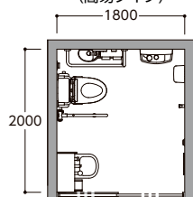
パリアフリートイレプラン例② (簡易タイプ)
