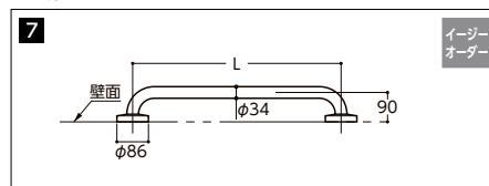
T112C6#NW1 希望小売価格 ¥17,500 長さ:600mm 握り径:φ34mm 抗菌
