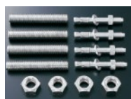
埋め込みセット T110D51 希望小売価格 ¥2,500 長ねじボルト(M10×60):4本 アンカーボルト(M6×50):4本 ナット:4個
