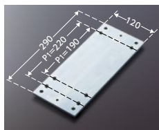
取付プレート 【パブリック用手すり はね上げ手すり(T112H型・T113H型・T114H型)、はね上げ手すり(EWC73型)用】 T110D49R 希望小売価格 ¥5,550 ※パブリック用手すり はね上げ手すりはP 1 =220、はね上げ手すりはP 1 =190の穴を使用します。 厚さ:6mm 1枚入り
