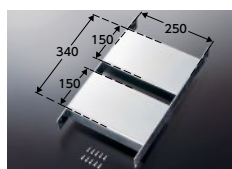
軽量鉄骨用取付金具 T110D36 希望小売価格 ¥15,500 取付金具(t3.2):1個 ドリルねじ(φ4×16):10本
