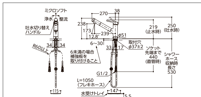
ホースが引き出せるハンドシャワー
