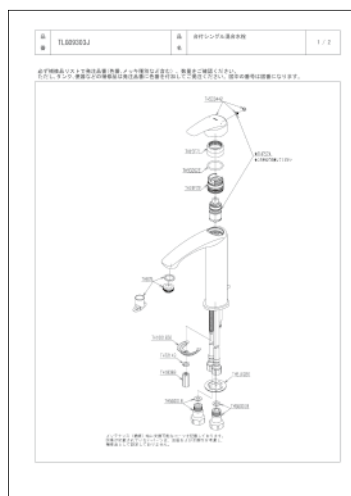
分解図
