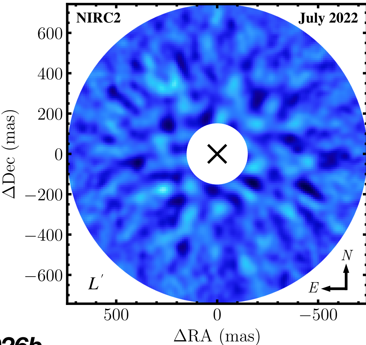
Keck / NIRC2 L' Imaging
