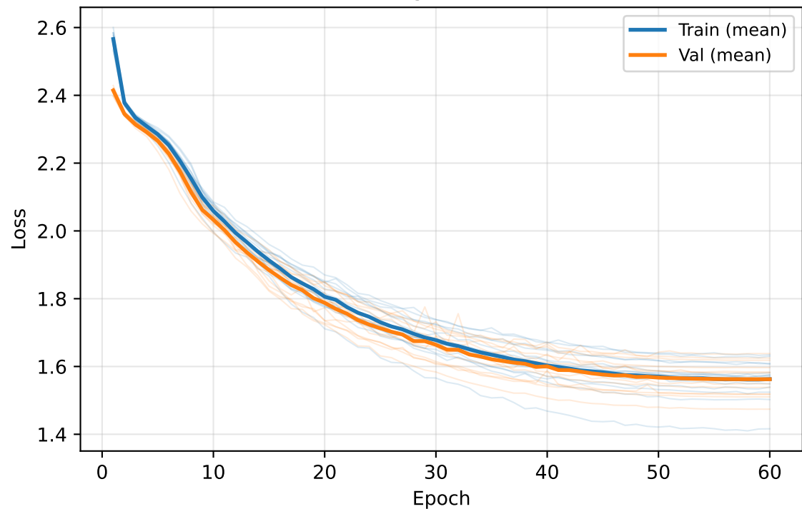
Stage 2 (KL)
