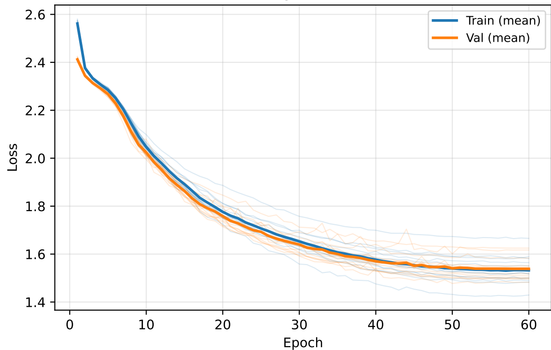
Stage 2 (KL)
