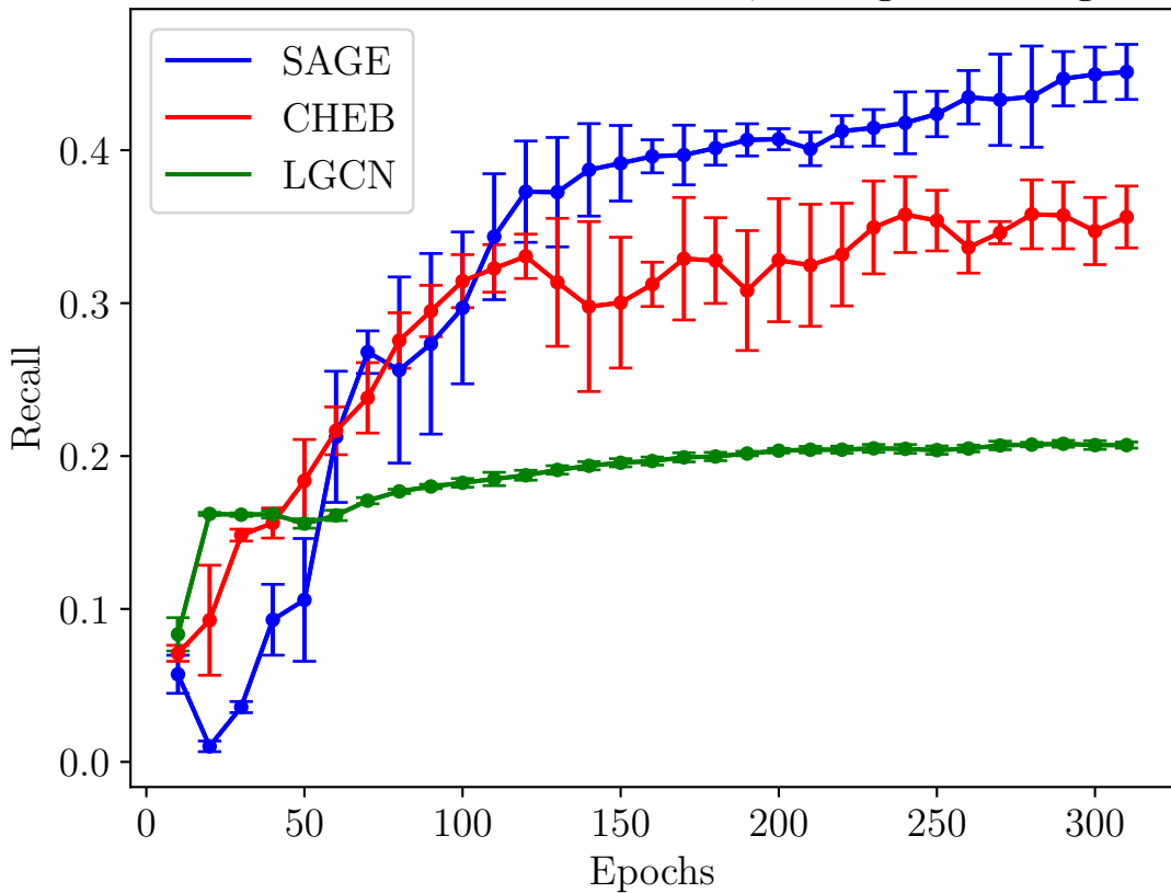
Amazon Data: Recall@392, 1 Negative Edge
