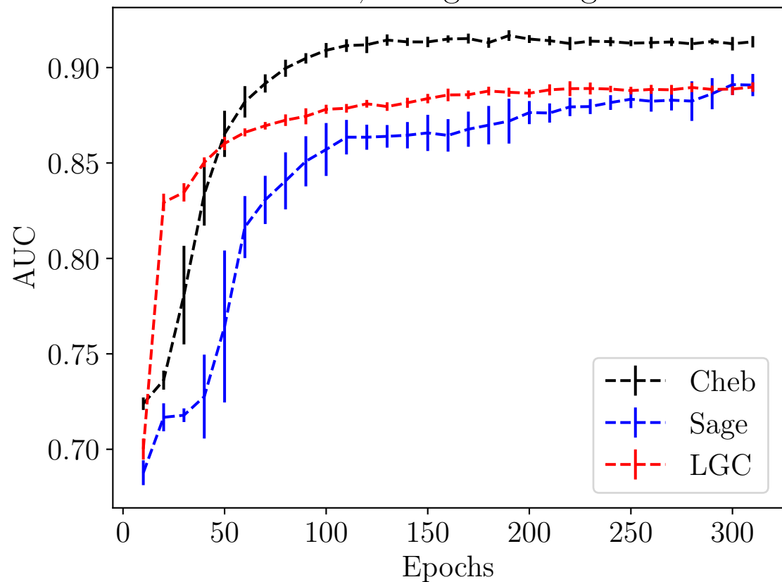
AUC, 1 Negative Edge
