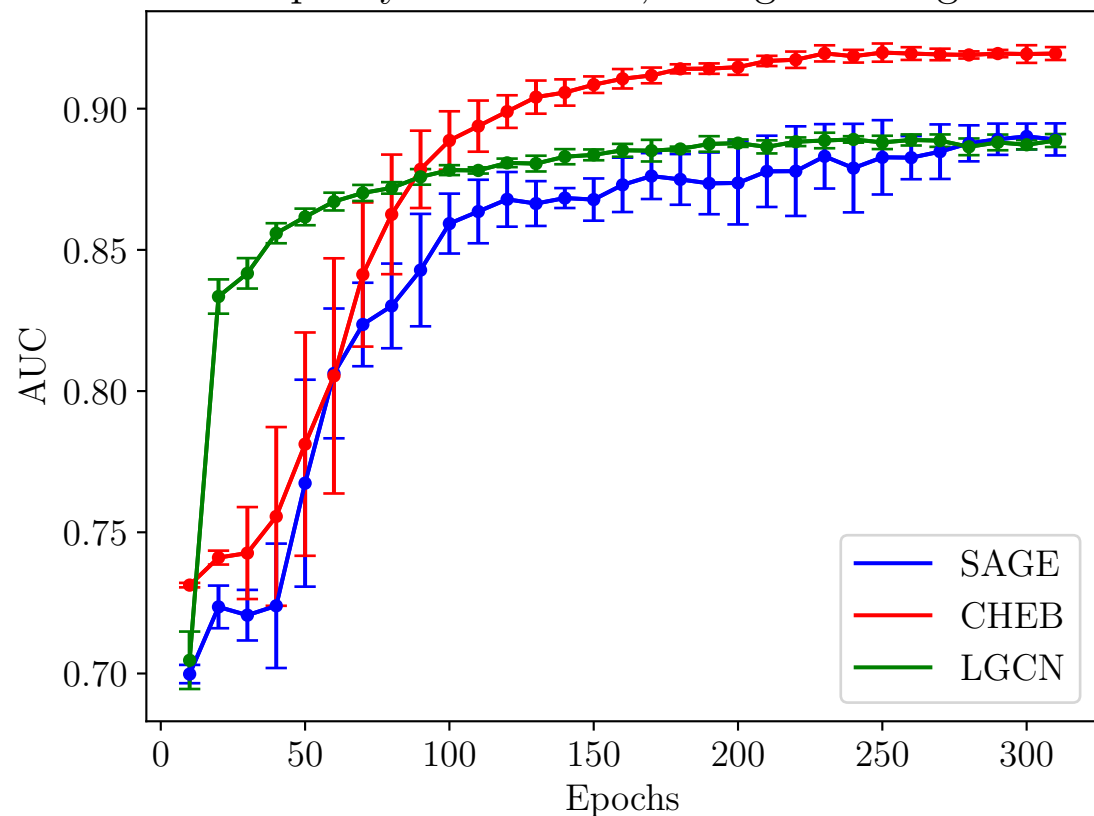
Spotify Data: AUC, 1 Negative Edge
