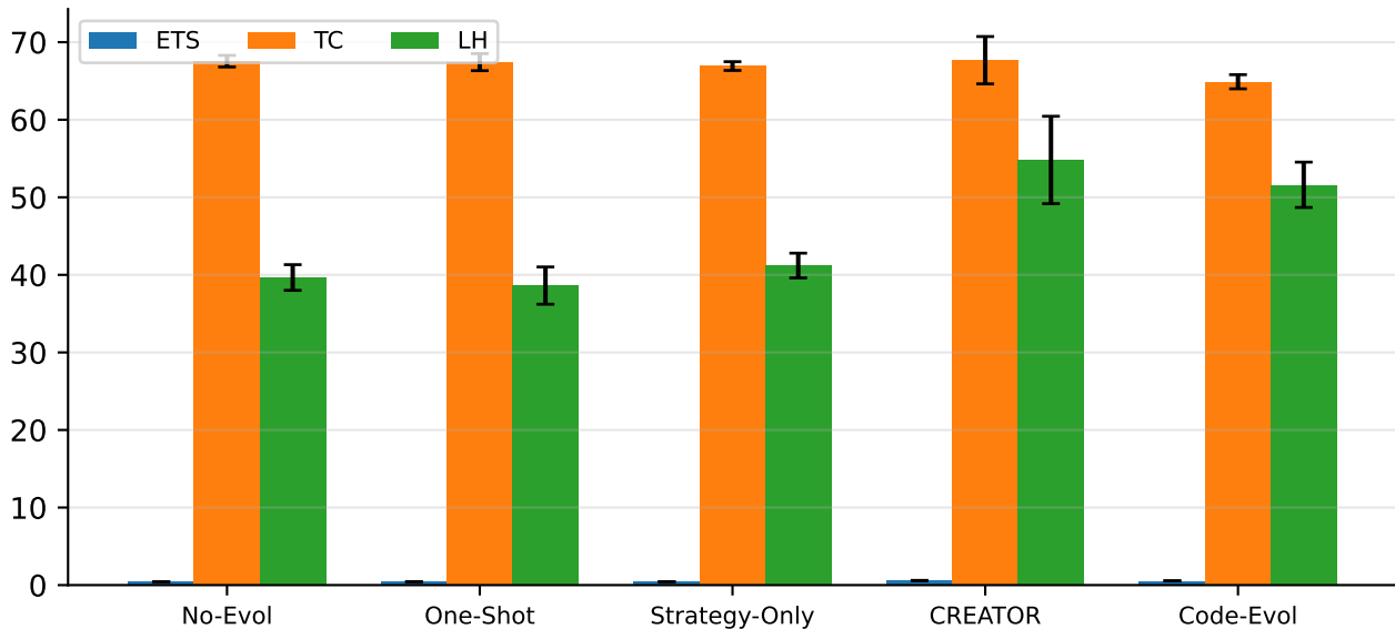
Score (ETS x100 scale)
