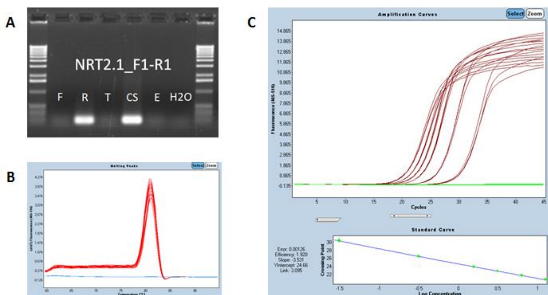
Figure 3-6 : Etapes de validation des couples d'amorces. Les couples sont testés par PCR sur des matrices d'ANDc issues de différents organes (A). Les matrices utilisées sont issues de feuilles (F), racines (R), tiges (T) et épis (E), et la PCR comprend également des témoins positif (CS) et négatifs (H2O). La spécificité des couples est ensuite validée plus formellement par l'analyse des courbes de dissociation en conditions de qRT-PCR (B). L'efficacité d'amplification des couples est enfin validée en qRT-PCR par la mesure d'efficacité d'amplification basée sur une gamme de matrices étalons d'ADNc (C).
