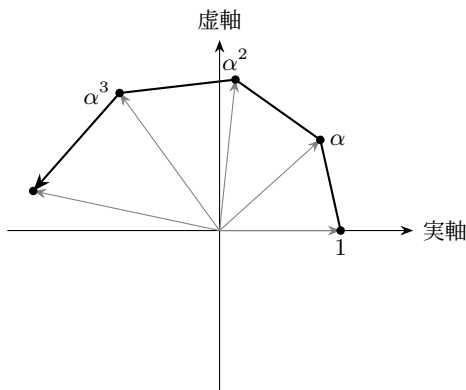
図 3.9 特性根の累乗は回転と伸縮の繰り返しになる
