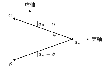
図 3.5 複素数の比は距離の比と偏角の差の両方を表す
