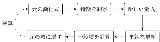
図 3.1 『きれいな形』へ帰着させるための一連の操作
