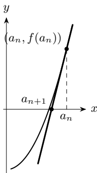
図 3.11 接線の x 軸との交点を次の近似値にする
