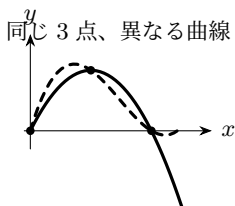
図 5.5 有限個の点を通る式は複数作れる
