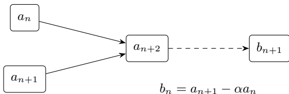
図 3.6 隣接 3 項間の更新には直前の二つの項が必要
