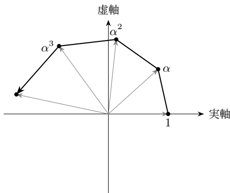
図 3.8 特性根の累乗は回転と伸縮の繰り返しになる
