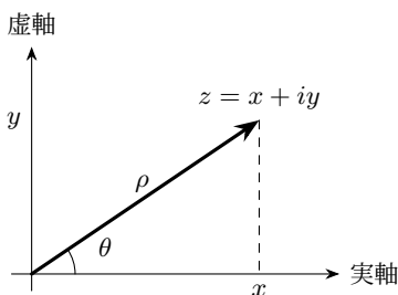
図 6.2 複素数を距離と偏角で表す
