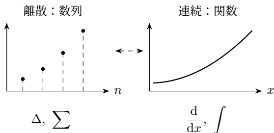
図 5.7 離散的な差分・総和と連続的な微分・積分
