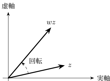
図 6.3 複素数の積は回転と伸縮を同時に表す
