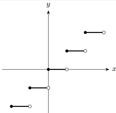
図 3.7 床関数は各整数区間で値が一定になる
