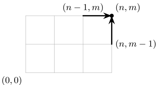
図 3.9 最後の一步で格子経路を二つに分ける
