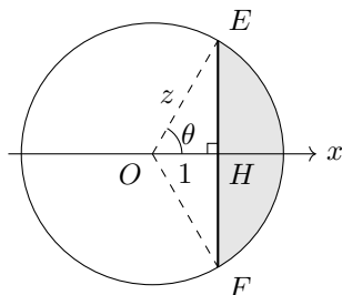
図 4.3 立体の水平断面と円弧・弦
