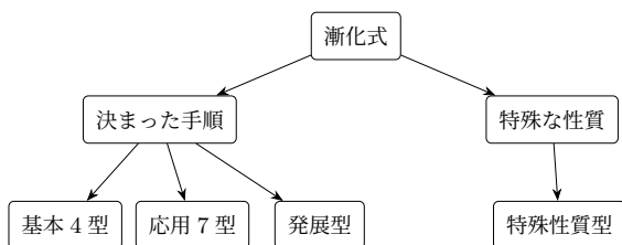
図 3.13 解法の系統と、それぞれの入口
