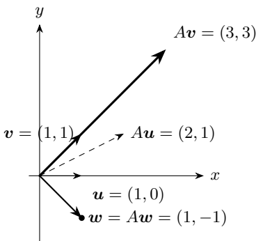
図 5.2 本文の行列 A では, 二つの方向がそれぞれ 3 倍と 1 倍になる
