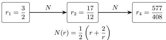
図 5.6 ニュートン法はペル解の添字を倍に進める
