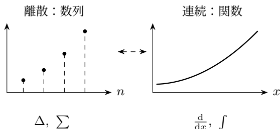
図 5.7 離散的な差分・総和と連続的な微分・積分
