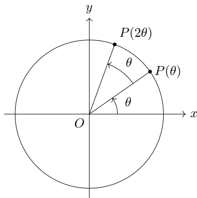
図 3.10 単位円における角度の倍化
