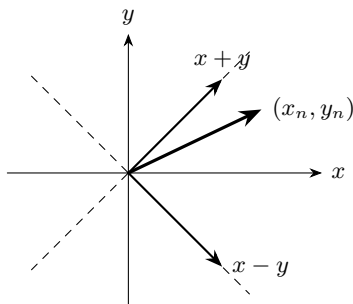
図 5.3 回転した座標軸では和と差が独立に更新される
