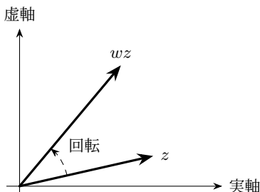
図 2.4 複素数の積は回転と伸縮を同時に表す
