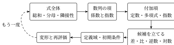
図 4.1 式全体・項・付加項の観察から解法候補を選ぶ
