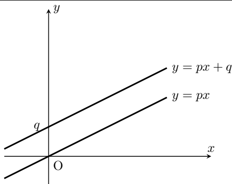
図 3.5 定数項の違いを表す平行な直線
