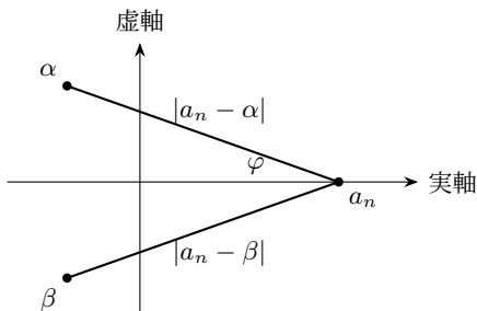
図 3.6 複素数の比は距離の比と偏角の差の両方を表す
