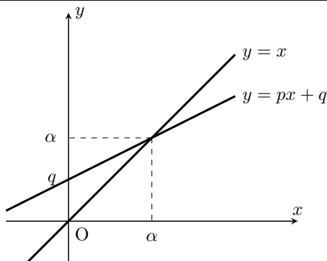
図 3.4 直線の交点として捉える不動点
