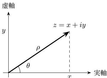
図 2.3 複素数を距離と偏角で表す
