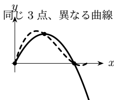
図 5.5 有限個の点を通る式は複数作れる 与えられた最初の N 項 a_1, \dots, a_N に対して,
