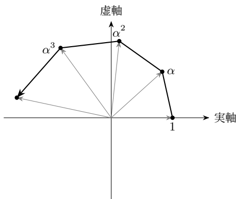
図 3.9 特性根の累乗は回転と伸縮の繰り返しになる
