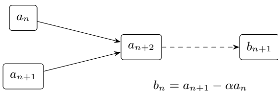
図 3.7 隣接3項間の更新には直前の二つの項が必要
