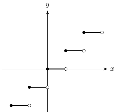
図 3.8 床関数は各整数区間で値が一定になる
