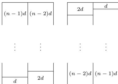
図 2.1 等差数列の増分を正順と逆順で組み合わせる
