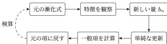
図 3.2 『きれいな形』へ帰着させるための一連の操作
