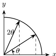
図 5.4 角の倍化とチェビシェフ多項式の対応
