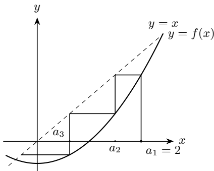
図 3.12 初項からの反復を y = f(x) と y = x で追う
