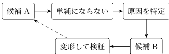
図 4.2 行き詰まりの理由を次の方針の手掛かりにする
