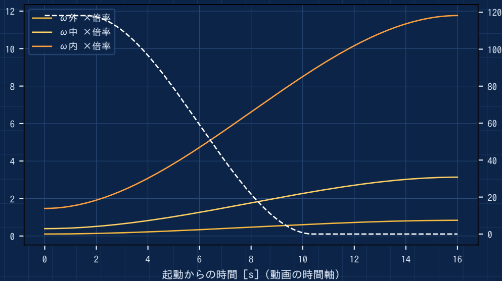
起動: 角速度 \omega(t) とポッド高度
