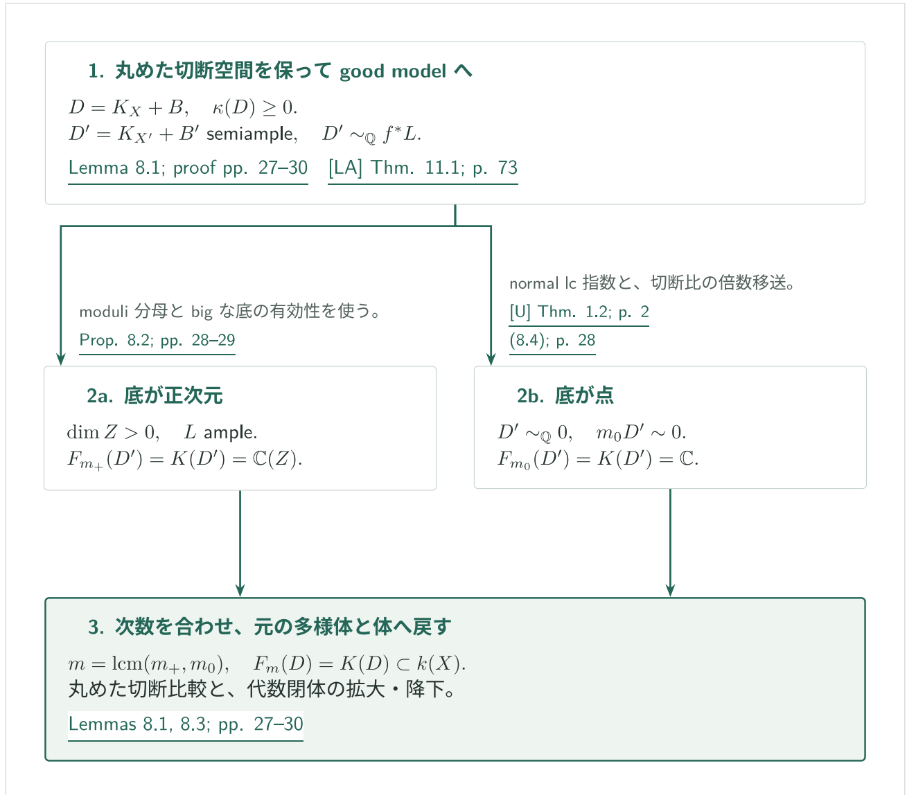
図4：good modelへ移り、正の飯高次元と0の場合を別々に処理して、元の体へ戻す。
