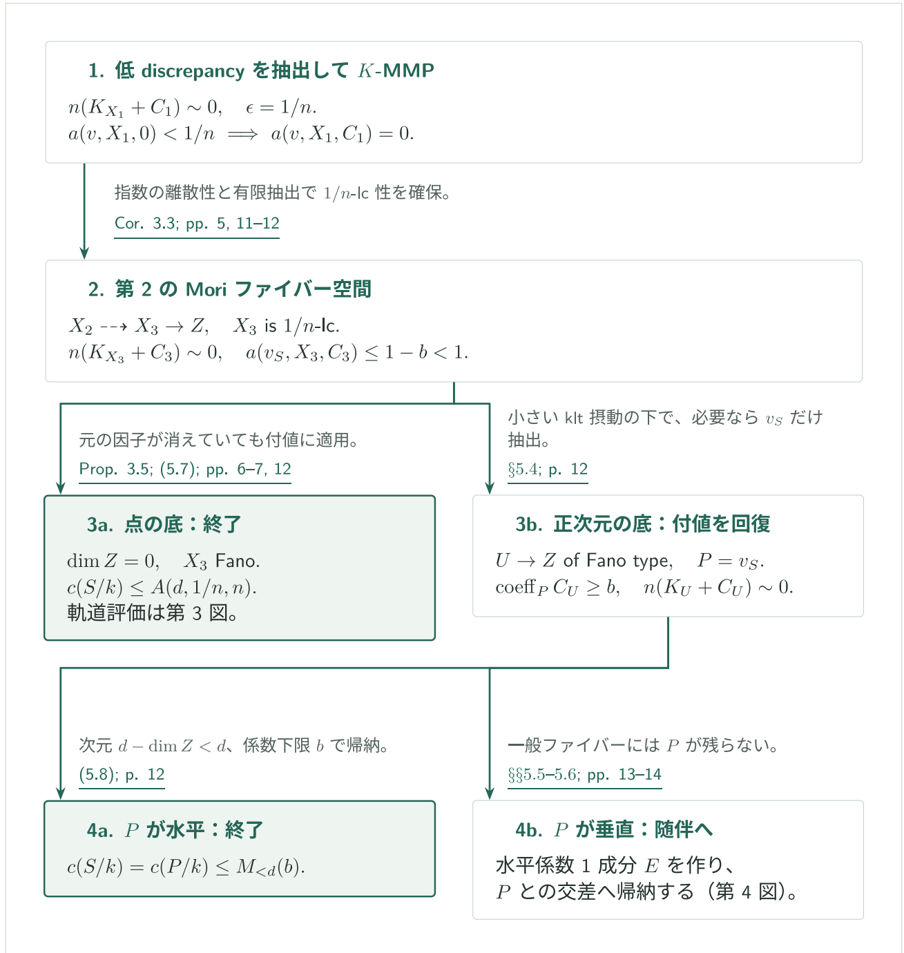
図2：第2のMMP。点の底はProposition 3.5、正次元の底では回復したPの水平・垂直で分岐する。
