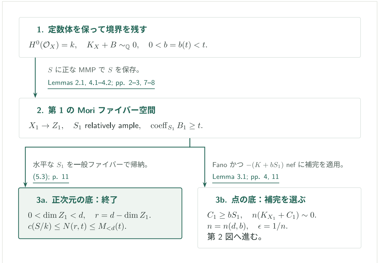
図1：最初のMMP。正次元の底では帰納法で終了し、点の底だけが補完と第2のMMPへ進む。
