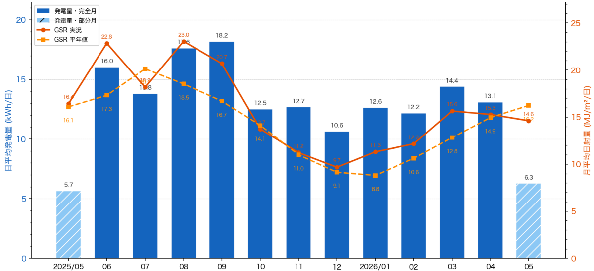
月別 日平均発電量・日射量 (2025/05~2026/05)
