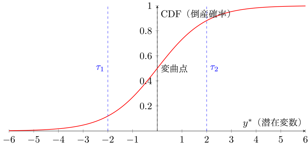
図 5.3: ロジスティック曲線の変曲点と閾値の概念図
