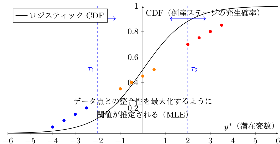
図 5.5: 閾値が尤度最大化 (MLE) によって推定される様子の概念図
