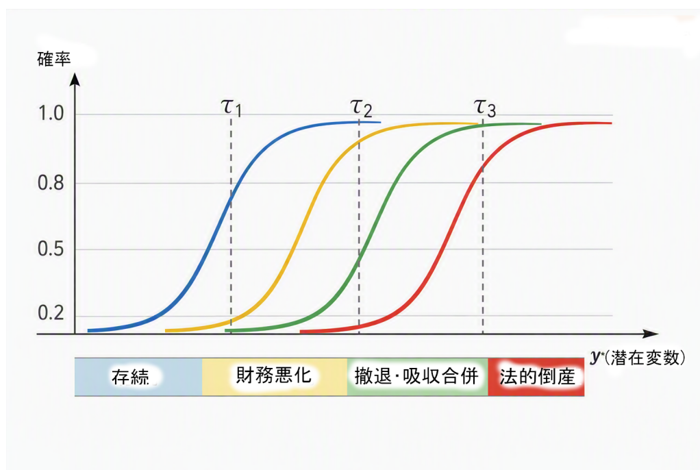
図 5.2: 閾値構造と倒産ステージの区分（概念図）
