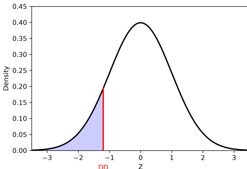
図 4.2: 標準正規分布における倒産距離 DD と倒産確率 \Phi(-DD)
